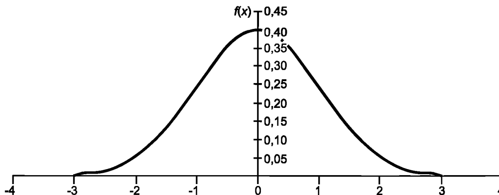
Рисунок Б.3 — Функция плотности нормального распределения
