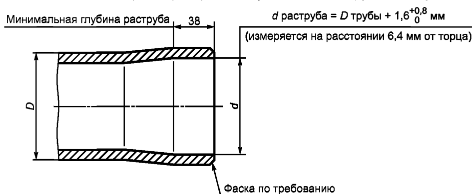
Рисунок 2 — Раструбный конец для соединения труб между собой
