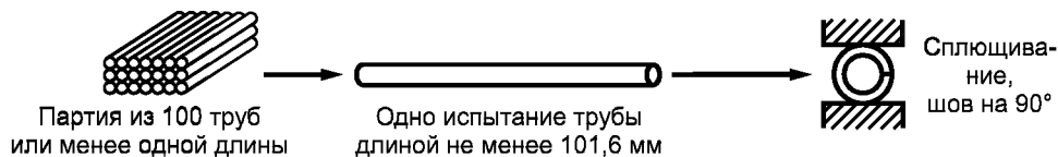
Рисунок 3 — Порядок отбора образцов для испытаний на сплющивание (8.5.1.2, 8.5.2.2).
