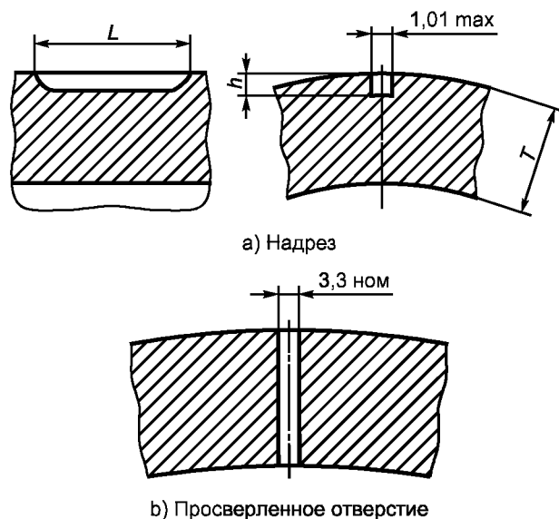
Рисунок D.1 — Эталонные образцы
