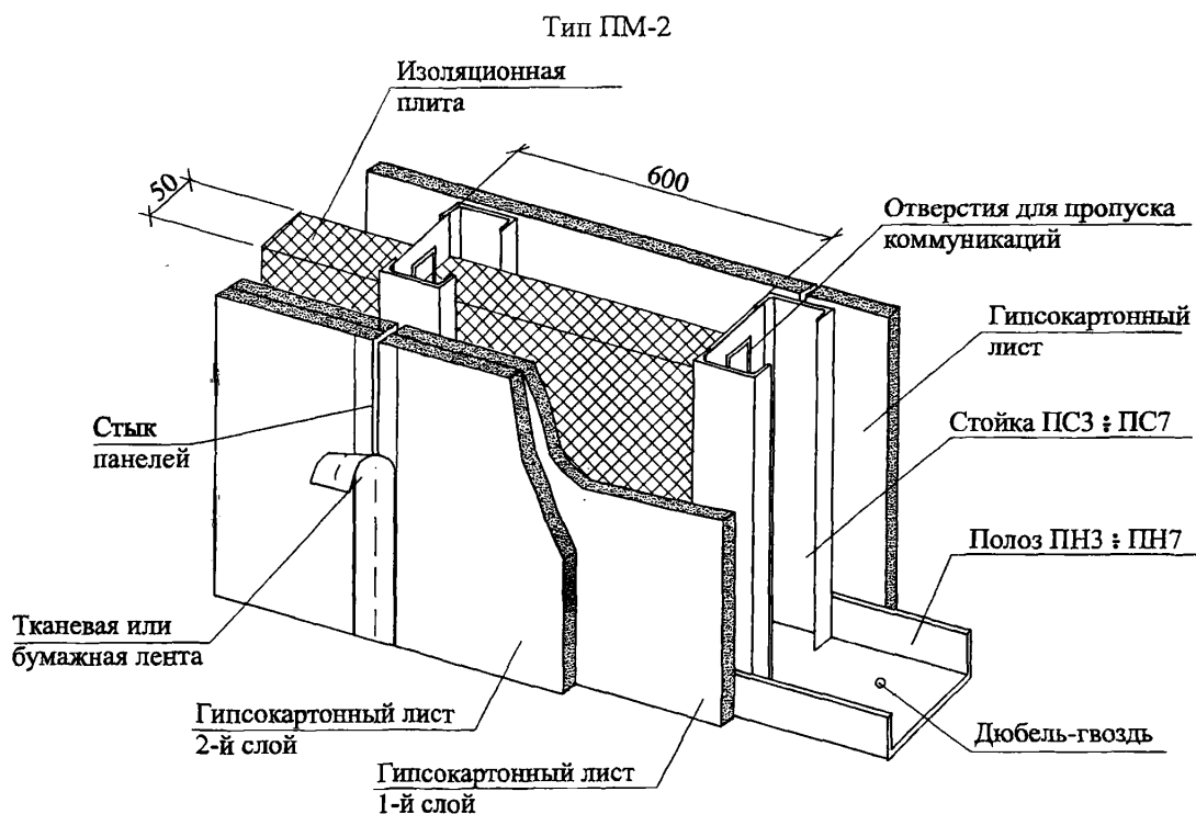
Рисунок 1 – Перегородки из гипсокартонных листов по металлическому каркасу
