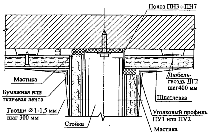
Г) Наружный и внутренний углы перегородки
