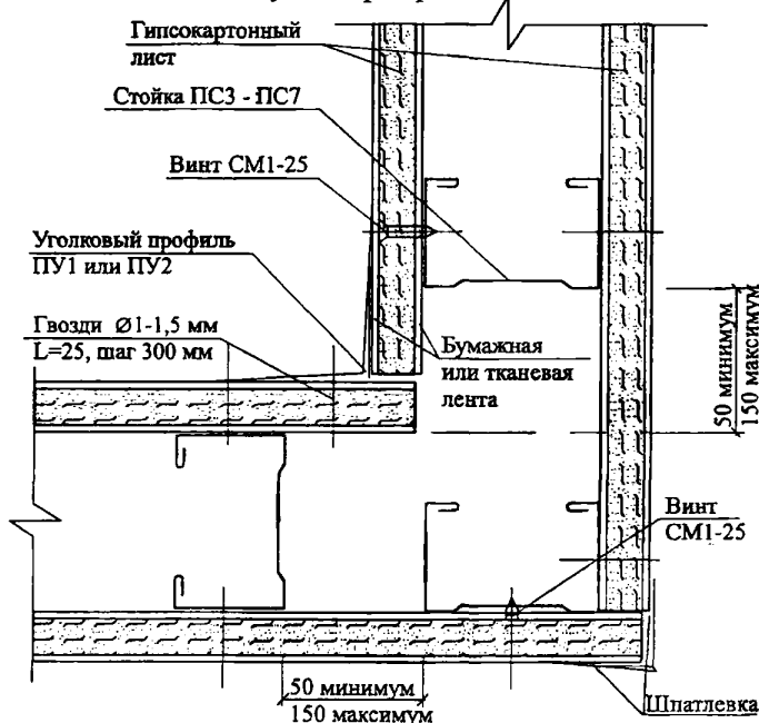
Д) Конструкция деформационных швов перегородки
