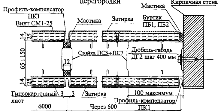
Рисунок 5 – Узлы примыкания перегородок
