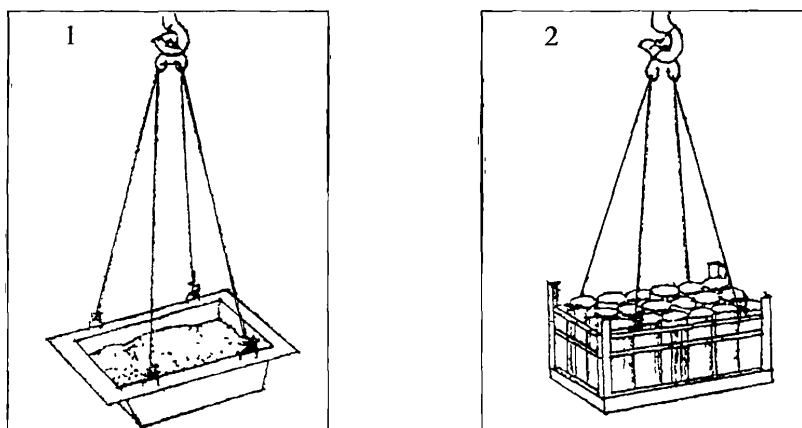
Рисунок 6 — Схемы строповок
