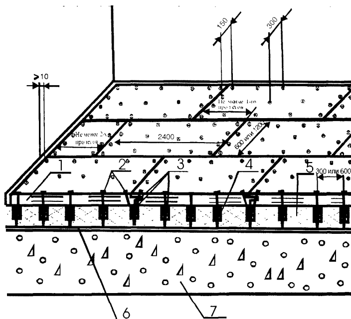
Рис. 3 Схема укладки древесностружечных плит в сборной стяжке опорах 1 - сборная стяжка из ДСП; 2 - гвоздь или шуруп; 3 - клей; 4 - регулируемые лаги; 5 - тепло-звукоизоляция из матов или плит; 6 - пароизоляция; 7 - железобетонная плита перекрытия
