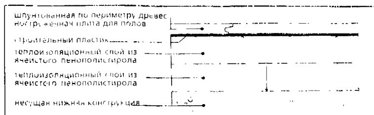
Рисунок 6. Использование строительного пластика между древесностружечной плитой и изоляционным слоем из ячеистого пенополистирола предотвращает появление неприятного скрипа.
