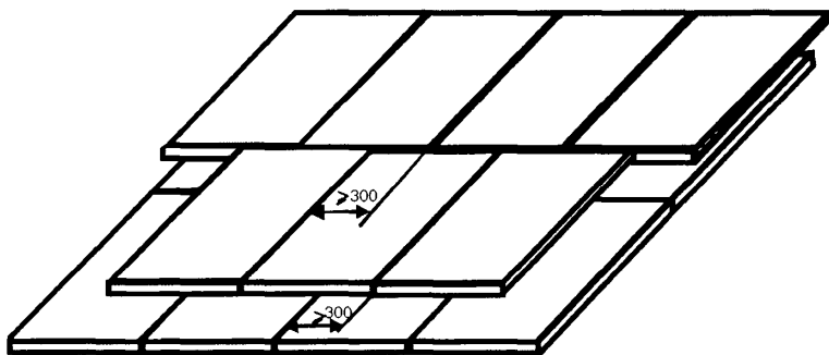
Рис. 2 Схема укладки тепло-звукоизолирующих пенополистирольных плит
