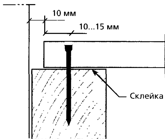
Рисунок 2. В пространстве у стен, проходов для трубопроводов и колонн предусматривается зазор размером не менее 10 мм.
