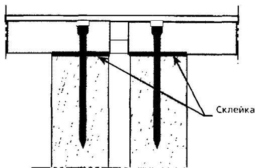
Шов расширения, например, под порогом или несущей перегородкой на полу на деревянных опорах
