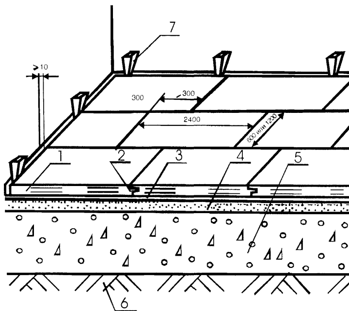
Рис. 3 Схема укладки древесностружечных плит в плавающей сборной стяжке 1 - сборная стяжка из ДСП; 2 - клеевая прослойка; 3 - пароизоляция; 4 - кварцевый песок; 5 - бетонное основание; 6 - грунт основания; 7 - клинья
