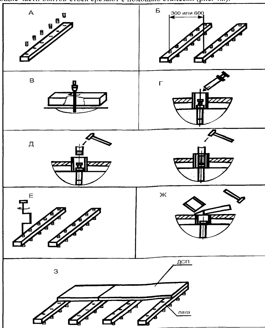
Рис. 4 Последовательные операции при установке регулируемых лаг и закреплении к ним сборной стяжки.
