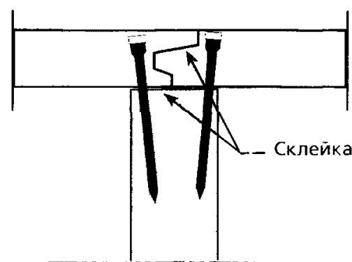
Рисунок 3. Крепление древесностружечной плиты в местах швов плит.
