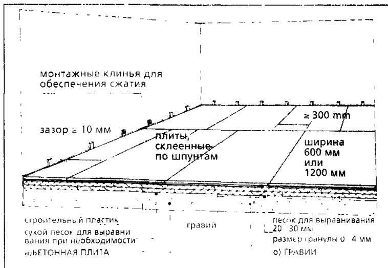
Рисунок 5. Монтаж плавающего древесностружечного пола а) на бетонной плите б) на слое из тщательно уплотненного и выровненного гравия. В качестве теплоизоляционного материала использован ячеистый пенополистирол.
