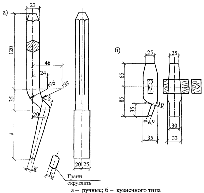
Рисунок 14 — Конопатки и чеканки.
