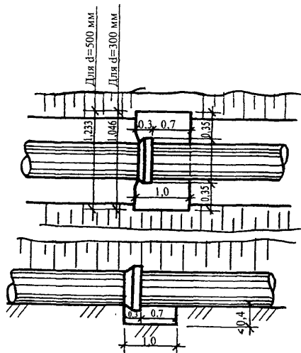
Рисунок 4 – Схема организации приямков
