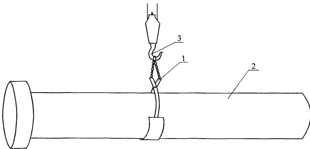
1 – клещевой захват; 2 – труба; 3 – гак подъемного механизма
