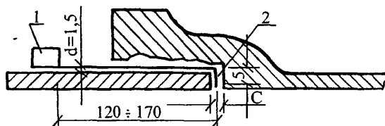
Рисунок 11 – Схема замера величины зазора между торцами стыкуемых труб
