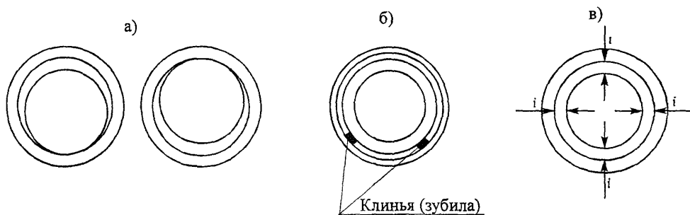
Рисунок 10 – Центровка труб со стороны гладкого конца (в раструбе уложенной трубы)
