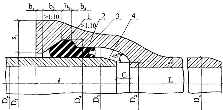
Рисунок 1- Раструбное соединение чугунных напорных труб (ТУ 14-3-1247-83) без устройства замка
