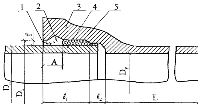
Рисунок 2 – Резиновая уплотнительная манжета (ТУ 38.105895-73).
