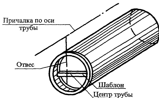
Рисунок 9 – Центровка труб со стороны раструба
