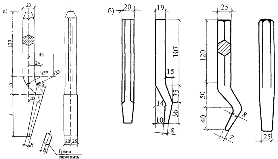
а – конопатка; б – чеканки
