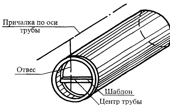
Рисунок 11 – Центровка труб со стороны раструба
