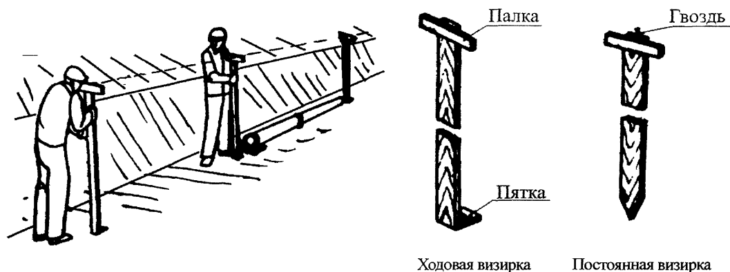
Рисунок 5 – Схема подготовки основания
