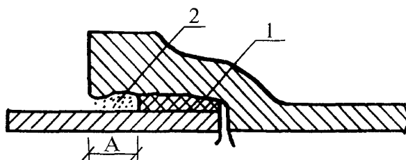
1 – уплотнение из пеньковой пряди, 2 – асбестоцементный замок (размер А); А = 35-40 мм для труб диаметром 65-400 мм
