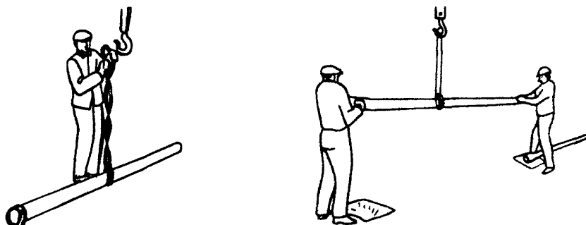
Рисунок 7 – Строповка труб и опускание в траншею
