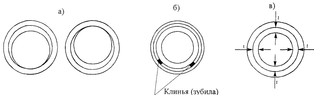
Рисунок 12 – Центровка труб со стороны гладкого конца (в раструбе уложенной трубы)
