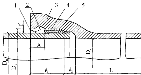
Рисунок 2 - Резиновая уплотнительная манжета (ТУ 38.105895-73).
