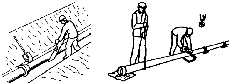
Рисунок 15 – Подбивка трубы грунтом и расстроповка трубы
