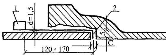
Рисунок 13 – Схема замера величины зазора между торцами стыкуемых труб
