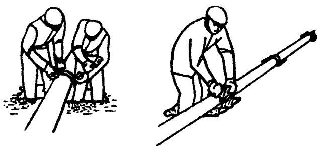
Рисунок 20 – Зачеканивание стыка
