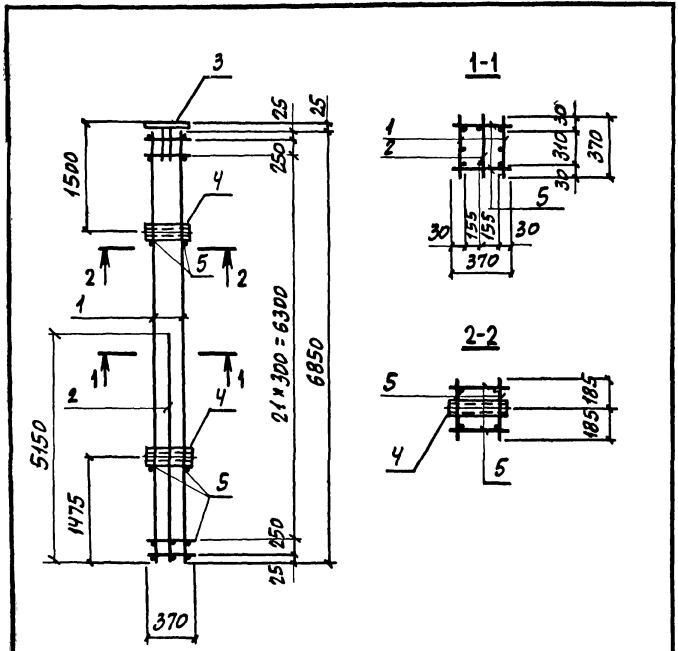
АРМАТУРА КЛАССА А-I по ГОСТ 5781-82
