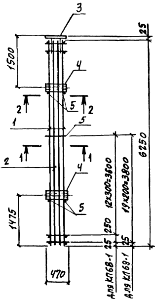
Арматура класса А-III по ГОСТ 5781-82
