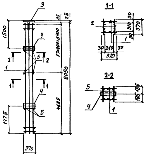
Арматура класса А-I по ГОСТ 5781-82
