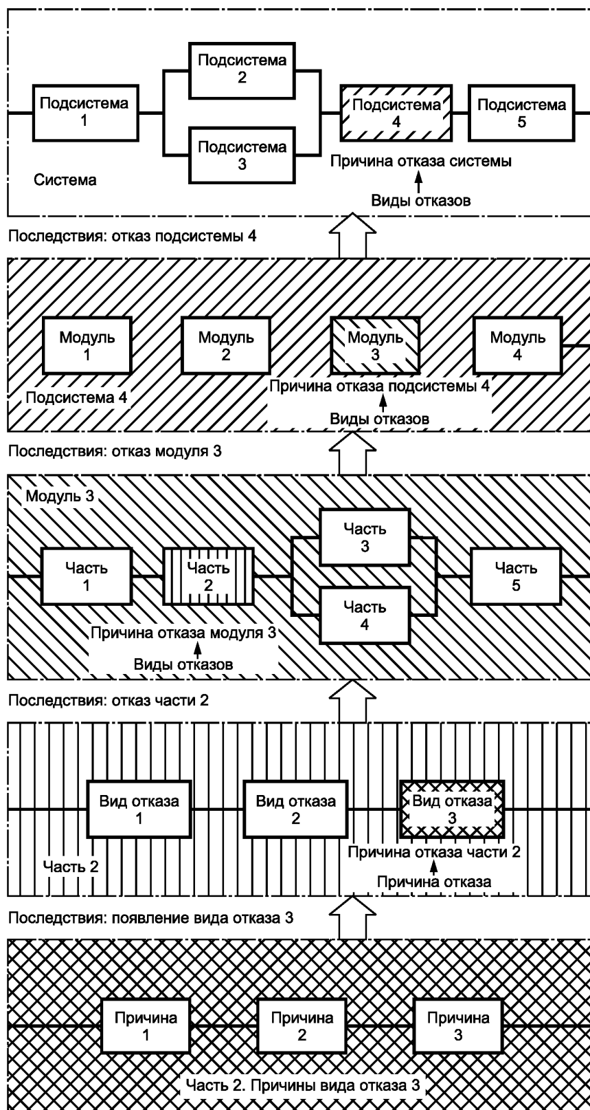
Рисунок 1 — Взаимосвязь видов и последствий отказов в иерархической структуре системы
