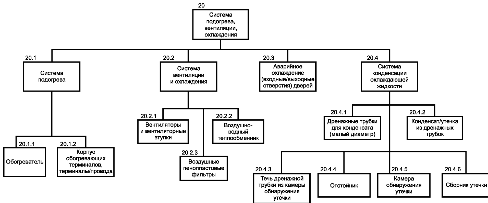
Рисунок В.3 — Диаграмма системы нагрева, вентиляции, охлаждения
