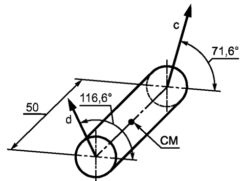
д) Векторы дисбалансов в торцевых плоскостях ротора
