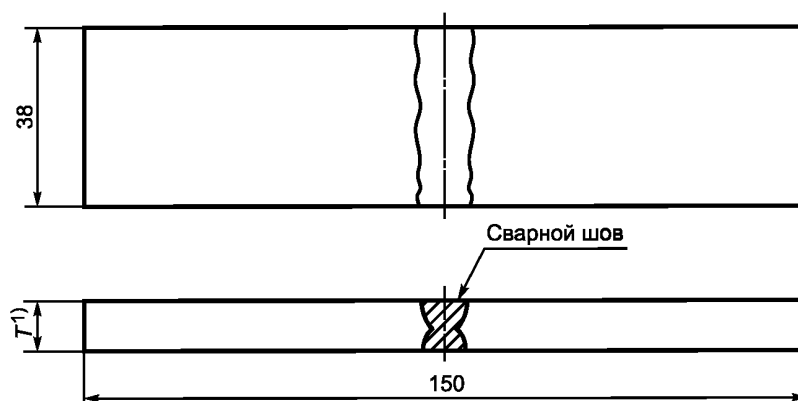
Рисунок 6 — Образец для испытания на изгиб
