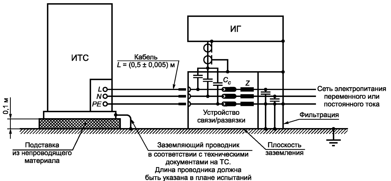
Рисунок 8 — Пример установки для испытания оборудования в стойке
