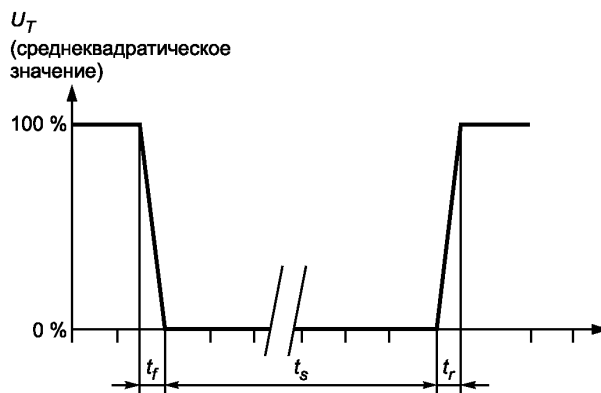
Рисунок 2 — Кратковременное прерывание напряжения
