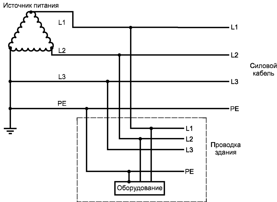
Заземленный проводник фазы
