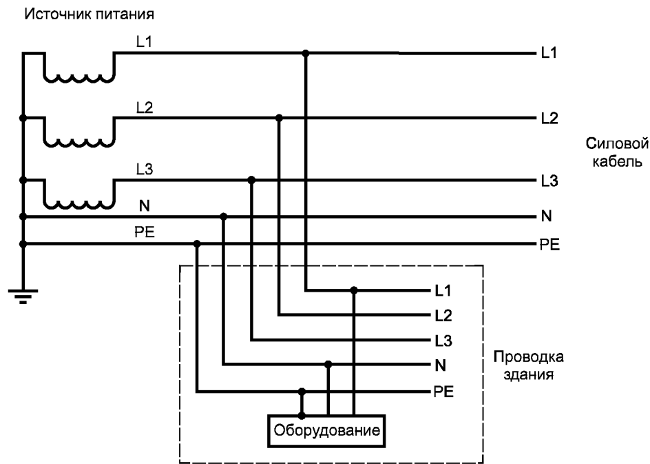
Разделенные нейтральный и защитный провода
