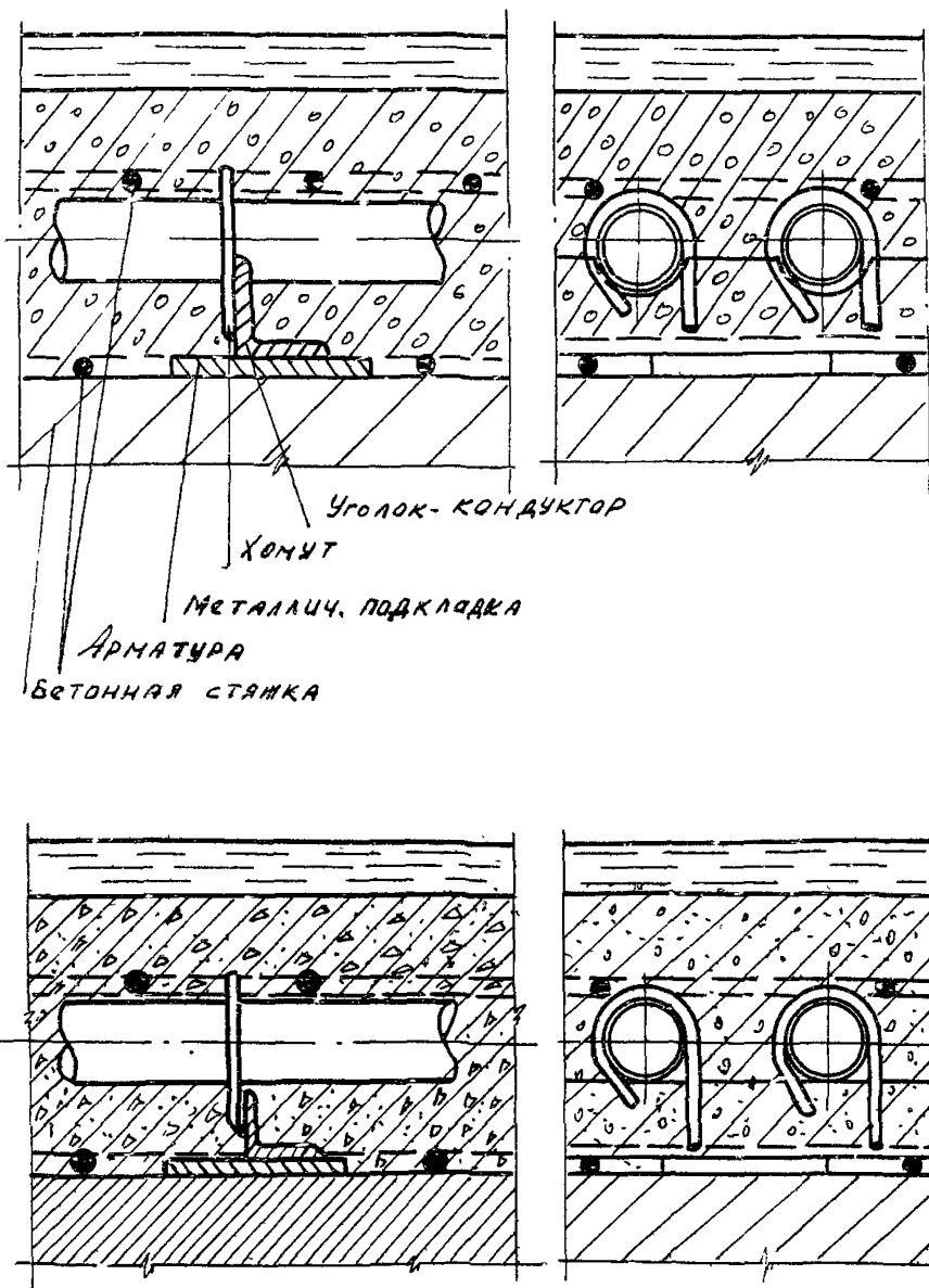
Рис. 15. Опоры для крепления труб в охлаждающей плите
