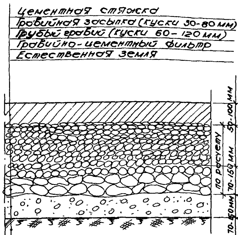
Рис. 11. Основание поля из крупноскелетных пород
