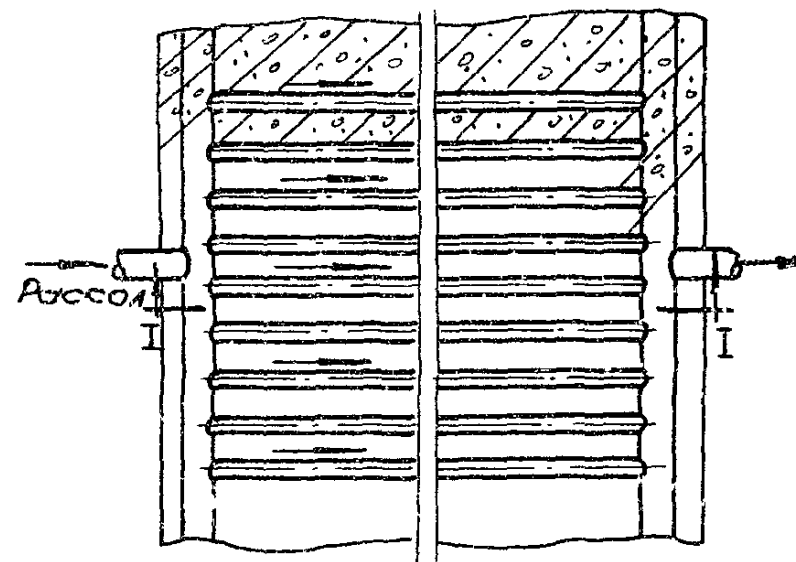
Рис. 18. Схема укладки труб с наклонным их расположением
