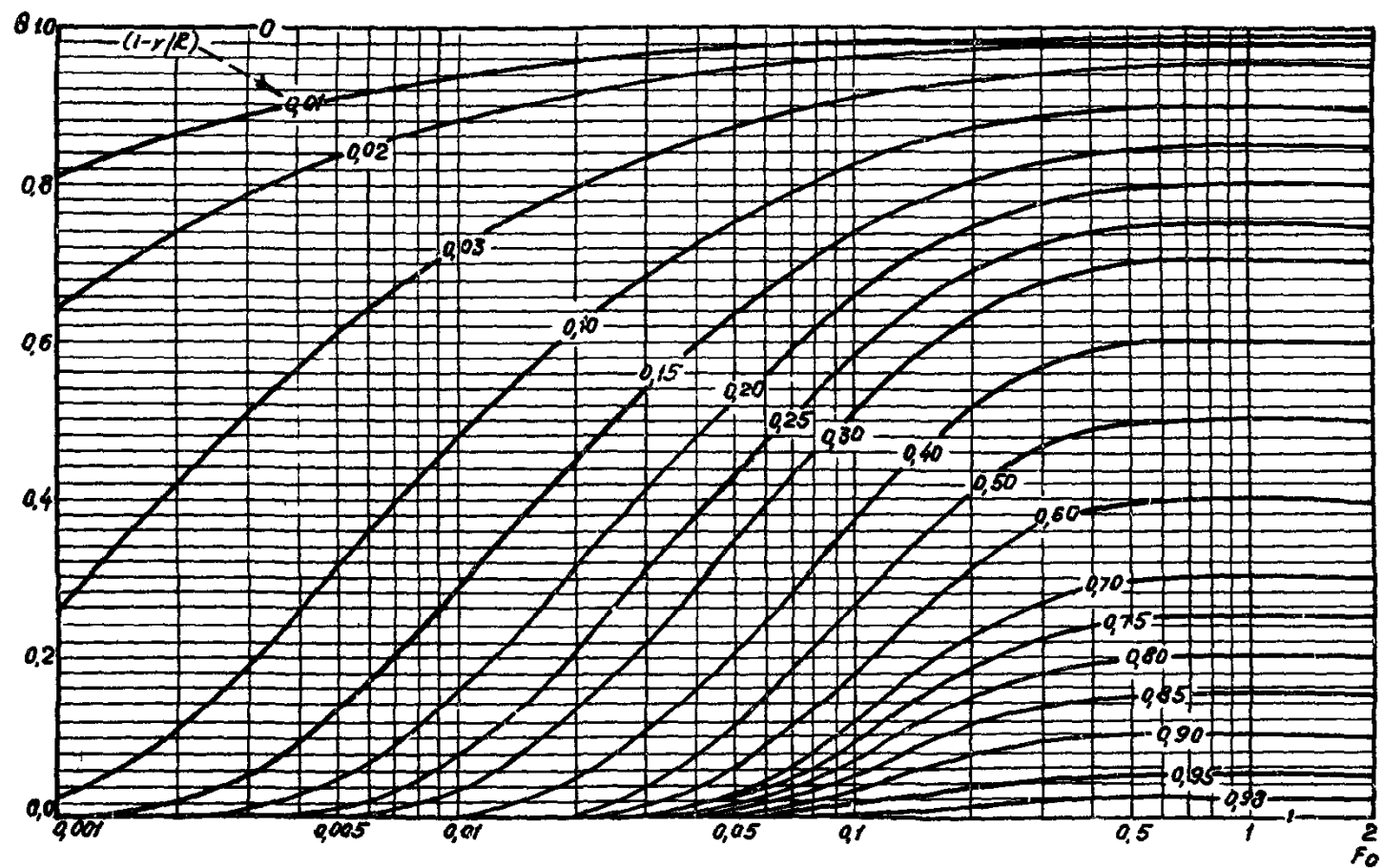
Рис. 10. Зависимость между Fo и \theta для пластины
