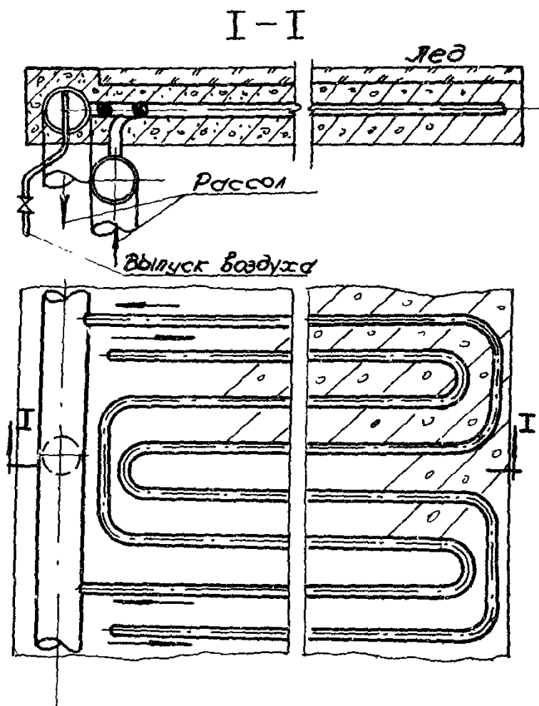
Рис. 16. Змеевиковая схема укладки труб
