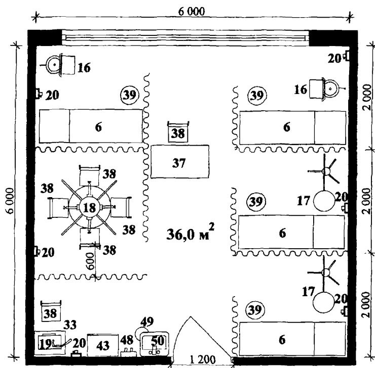
Рис. 1.4. Кабинет электросветолечения на 6 аппаратов
