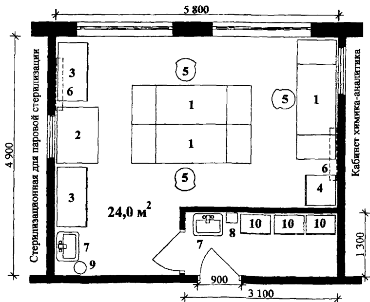
Рис. 2.1 Ассистентская-асептическая со шлюзом для больниц на 1000 коек
