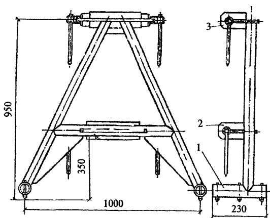
Рис. 7. Упор
