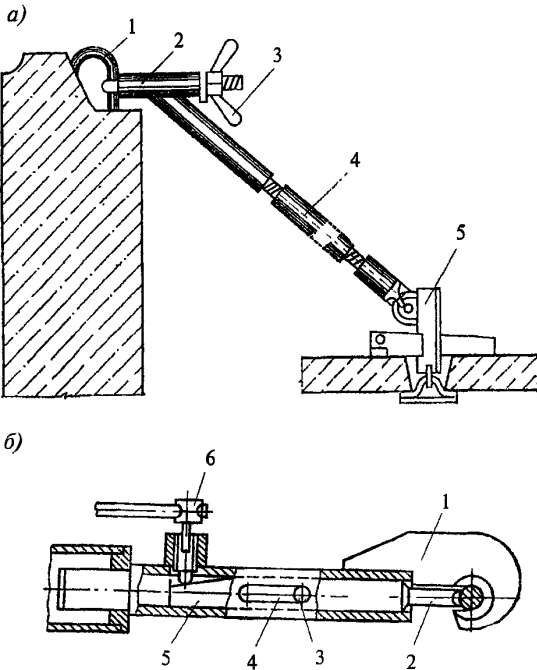
Рис. 4. Подкосы
