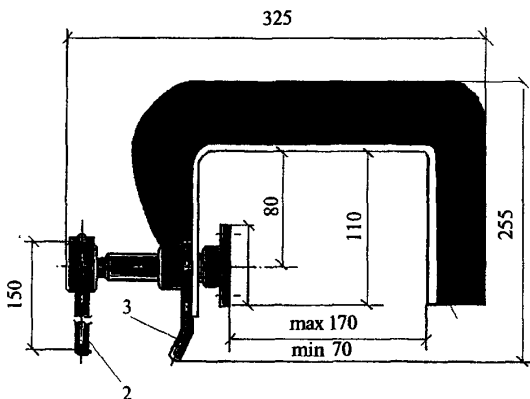
Рис. 2. Струбцина
