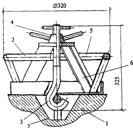
Рис. 3. Анкер
