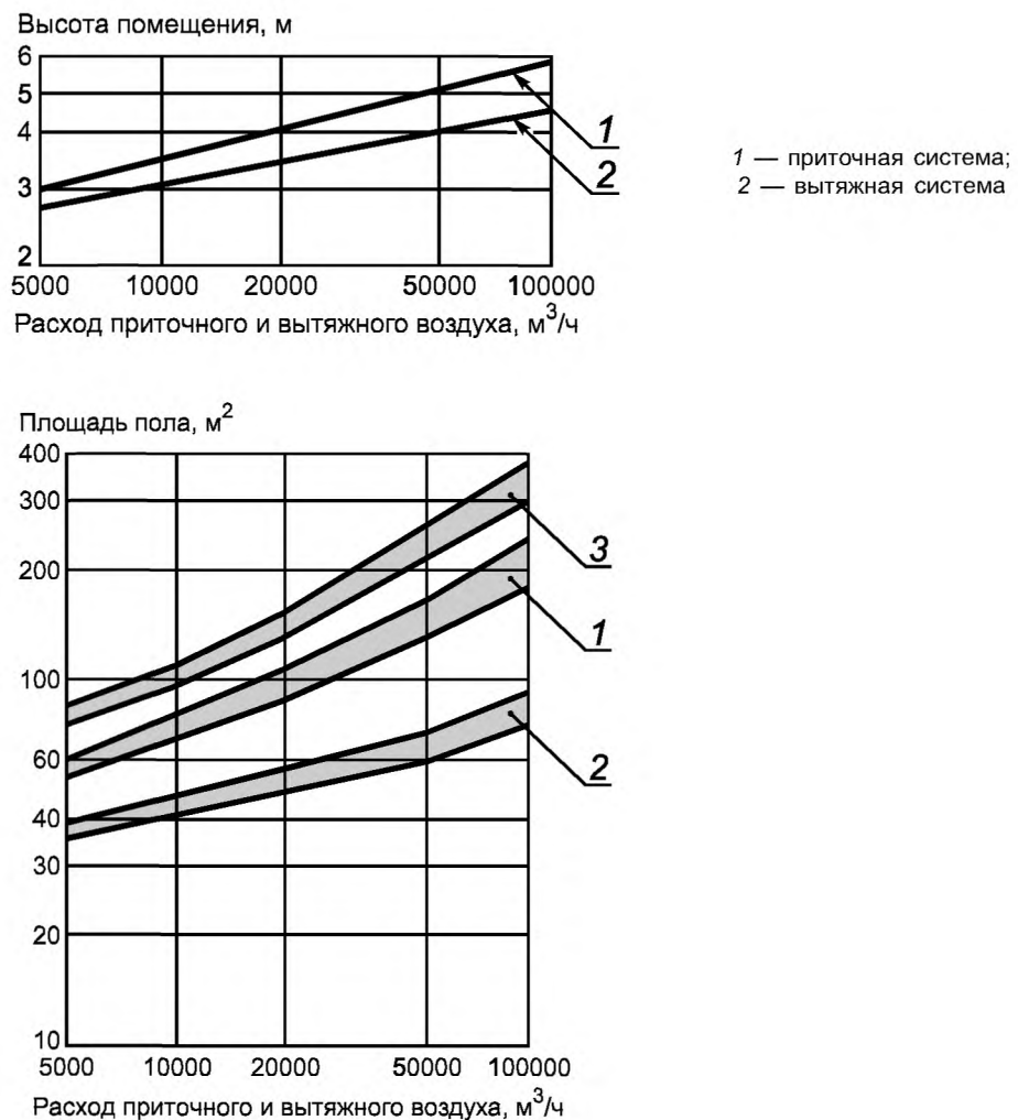
Рисунок А.4 — Высота и площадь вентиляционных камер
