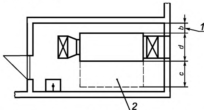
Рисунок А.5 — Расположение кондиционера (в плане)
