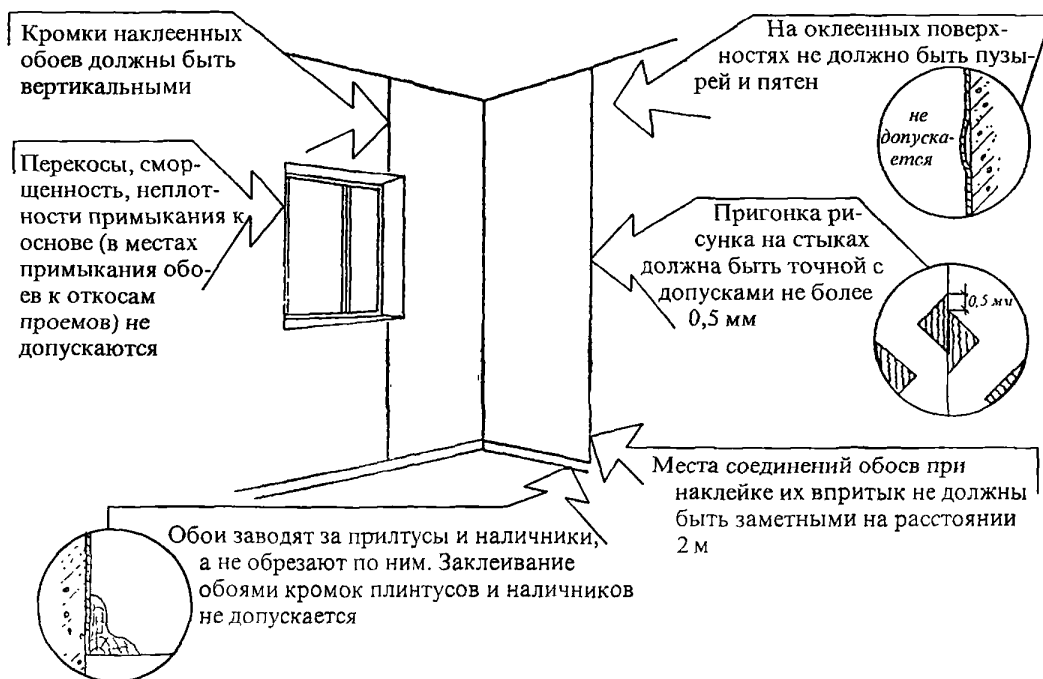
Рисунок 35 – Основные требования к обойным работам
