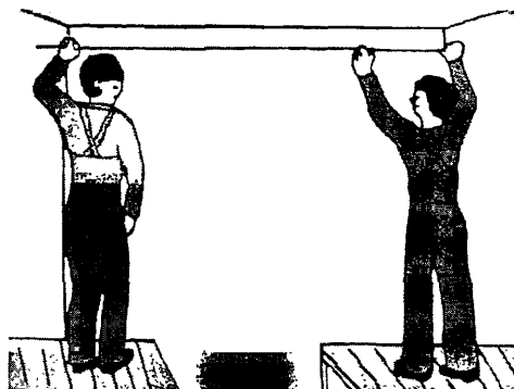
Рисунок 1 – Разбивка линии верха обоев наметленным шнуром
