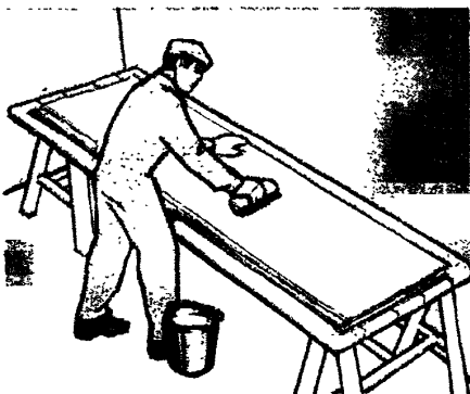
Рисунок 11 – Нанесение клейстера на полотнища
