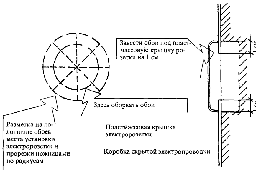
Рисунок 17 – Обработка мест примыкания обоев к электророзеткам
