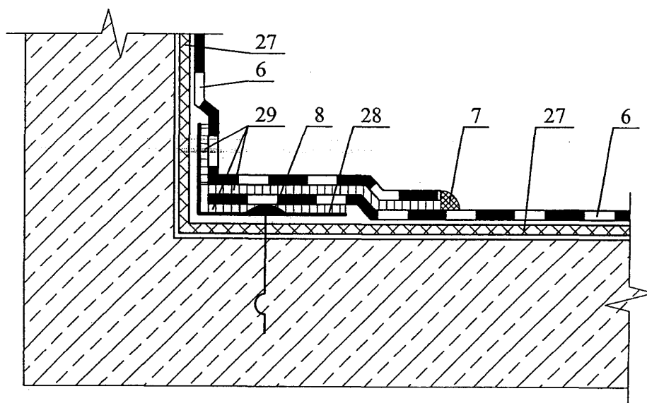
Узел 1.2 - 1
