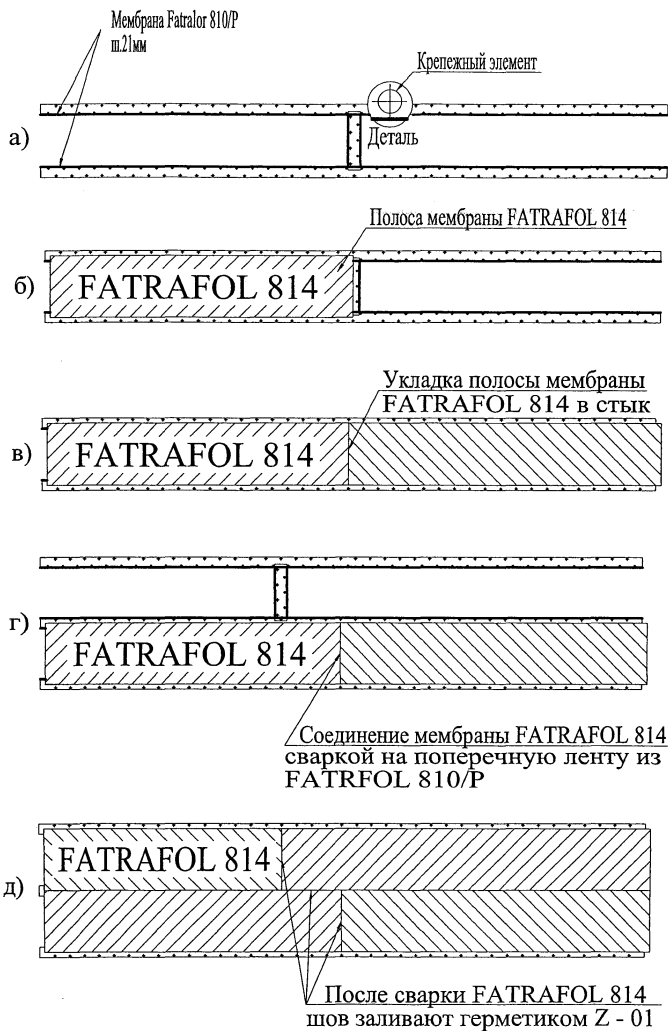
Рис. 4. Укладка мембраны Fatrafol 814
