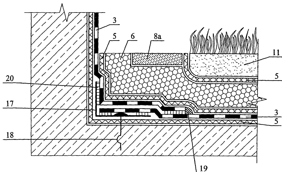
Узел 15.1 - 2
