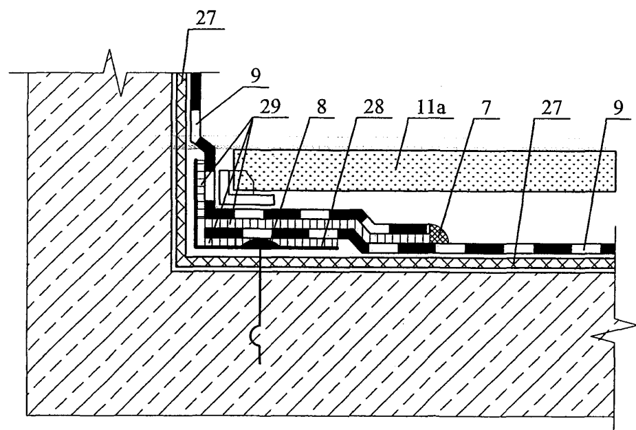
Узел 2.2 - 1
