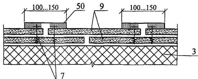
Узел "Б.1"
