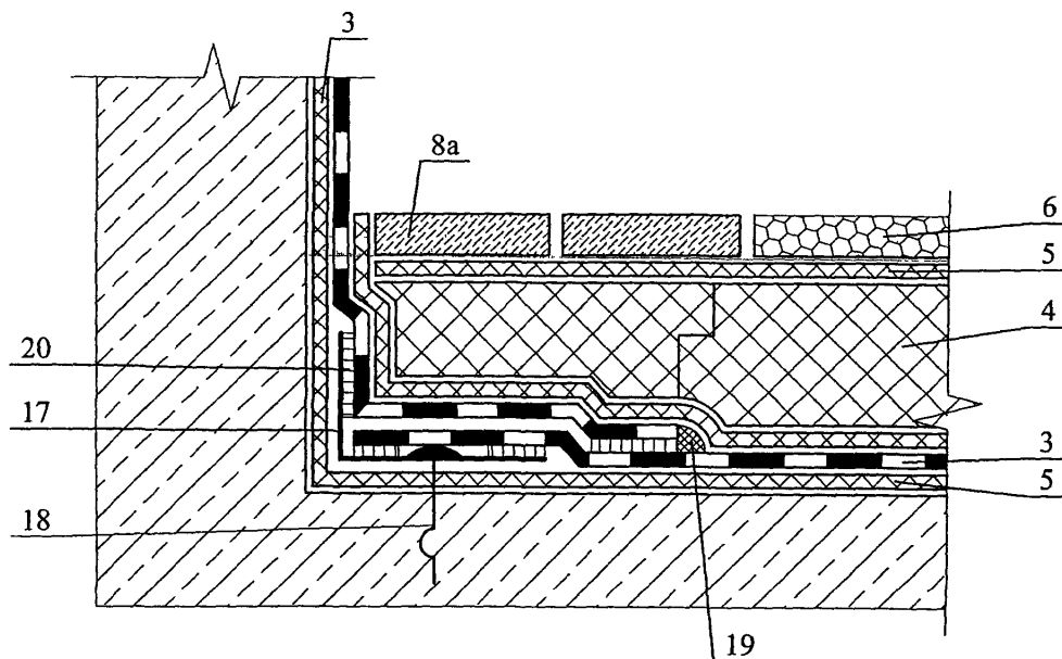
Узел 15.1 - 1
