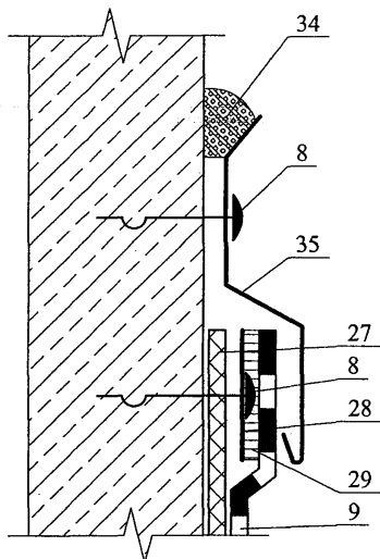
Узел 2.1 - 1
