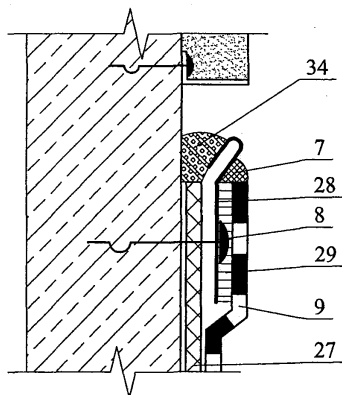
Узел 2.1 - 3
