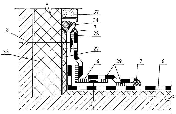
Узел 1.2 - 5
