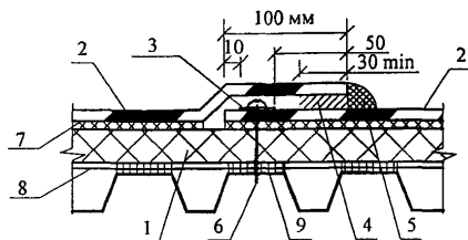
Рис. 2. Стык смежных полотен рулонного материала
