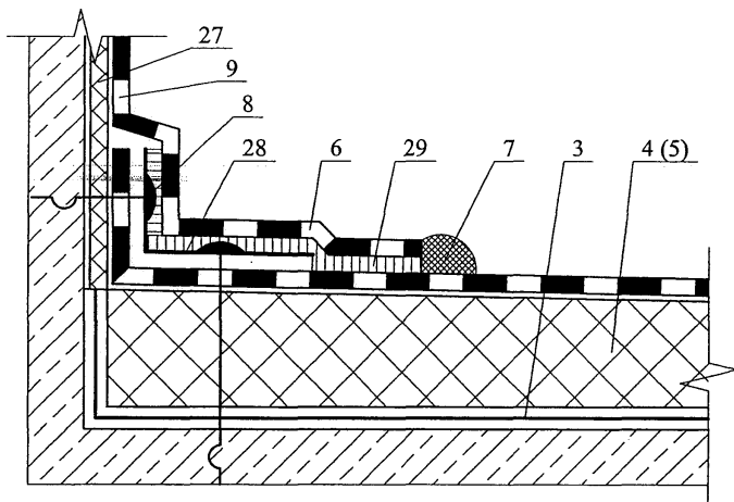
Узел 1.2 - 3
