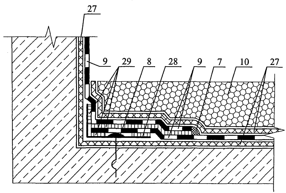
Узел 2.2 - 2
