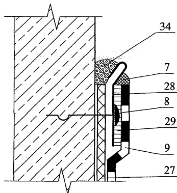
Узел 2.1 - 2
