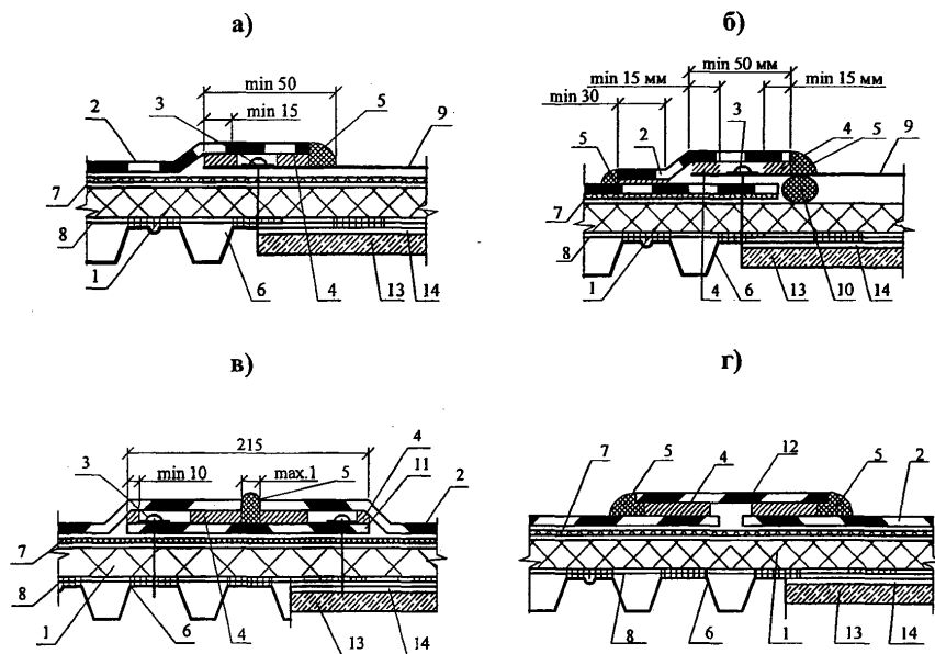
Рис. 3. Соединение
