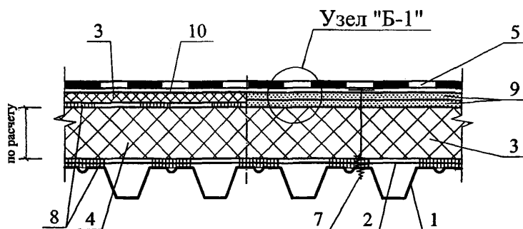
Узел "Б.1"
