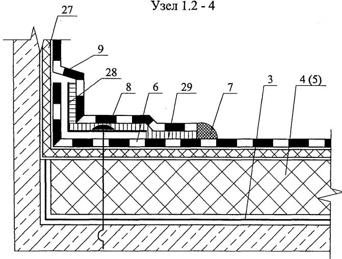
Узел 1.2 - 4
