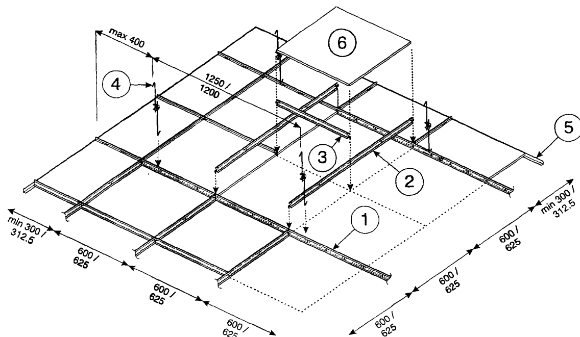
1 – несущая рейка; 2 – поперечная рейка; 3 – поперечная рейка; 4 – подвес; 5 – стенной молдинг; 6 – плита
