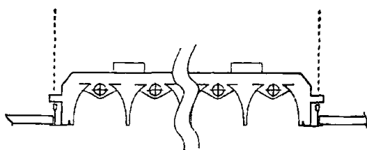
Универсальная несущая рейка Prelude 24
