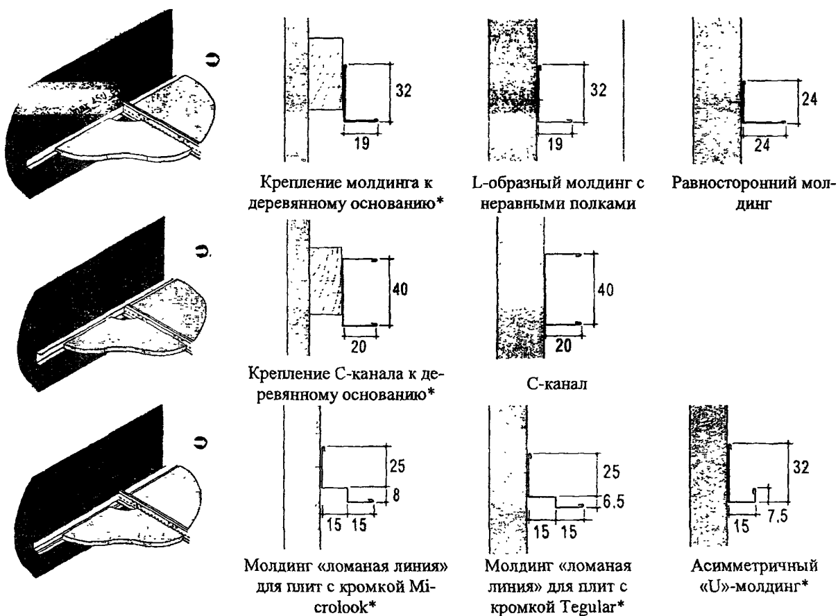
Рисунок 21 – Различные варианты стенных молдингов
