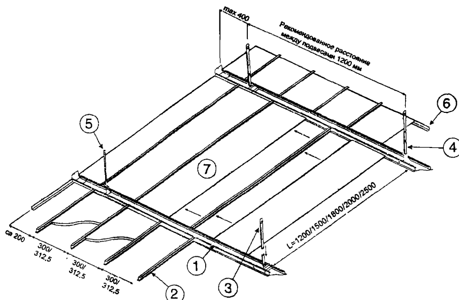
Рисунок 19 – Схема монтажа подвесных потолков «Армстронг» Prima Planks на полускрытой системе SL2/K2C2 (несущие рейки Trulok 24 или Bandraster)
