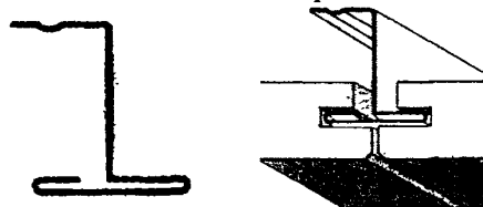
Рисунок 11 – Подвесные системы и типы кромок потолочной плиты «Армстронг»
