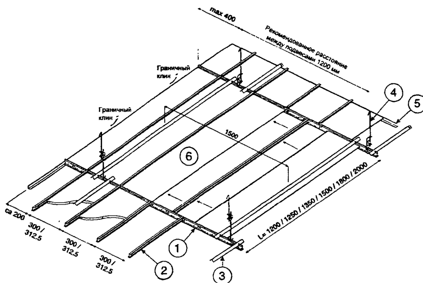
Демонтаж планок
