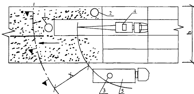
Рисунок 3 – Схема организации рабочего места при устройстве песчаного подстилающего слоя
