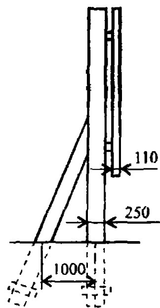
Рис. 7. Снегопередвигающие деревянные заборы (размеры даны в мм)
