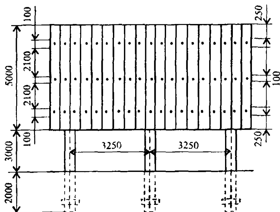
Рис. 7. Снегопередвигающие деревянные заборы (размеры даны в мм)
