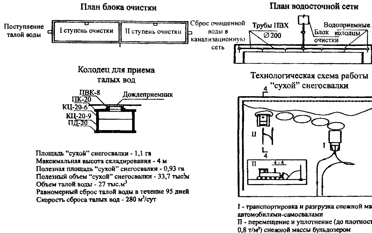
Рис. 17. Схема «сухой» снегосвалки
