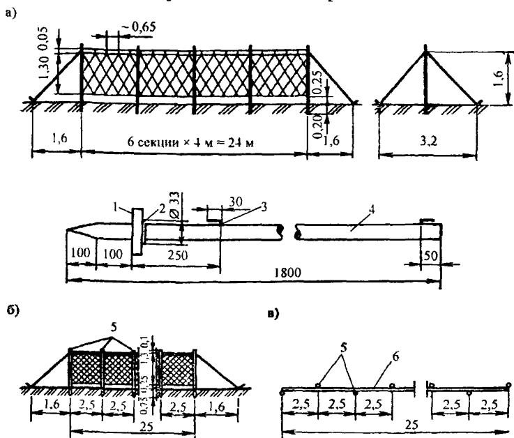
Рис. 13. Снегозадерживающие полиэтиленовые сетки: а – тип I на стойках металлических труб; б – тип II на деревянных кольях; в – размещение кольев; 1 – стопорная шайба \varnothing 150 \times 5 с отверстием \varnothing 33 мм; 2 – упор; 3 – крепление для сетки \varnothing 5 мм; 4 – стальная труба \varnothing 33 - 24 мм; 5 – деревянные колья \varnothing 80-100 мм; 6 – сетка
