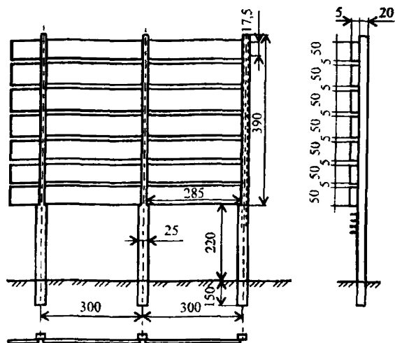
Рис. 8. Снегопередующий керамзитобетонный забор (размеры даны в см)
