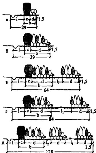
Рис. 4. Типовые схемы усиления существующих снегозащитных лесных насаждений вдоль автомобильных дорог при объеме снегоприноса ( \text{м}^3/\text{м} ): a — до 25; б — до 50; в — до 100; г — до 150; д — до 250
