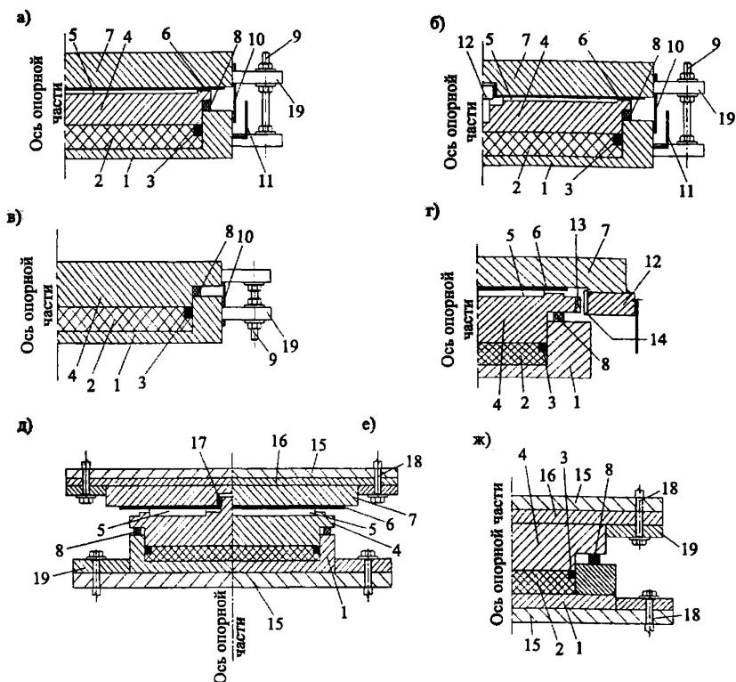
Рис. 10. Конструкции стаканных опорных частей: а — всесторонне-подвижная; б — линейно-подвижная с направляющими элементами в середине крышки; в — неподвижная; г — линейно-подвижная с направляющими элементами с наружных сторон крышки; д, е, ж — линейно-подвижная, всесторонне-подвижная и неподвижная с элементами анкерного крепления; 1 — стакан; 2 — резиновая пластина; 3 — уплотнительные кольца; 4 — крышка; 5 — фторопластовая пластина; 6 — стальной полированный лист; 7 — скользящая плита; 8 — уплотнитель; 9 — транспортный болт; 10 — фартук; 11 — указатель перемещений; 12 — направляющая; 13 — фторопластовая или металлофторопластовая полоса; 14 — стальная полированная полоса направляющей; 15 — анкерная плита; 16 — прокладная плита; 17 — пара трения фторопласт или металлофторопласт — полированная сталь; 18 — анкерный болт; 19 — уши для транспортных болтов
