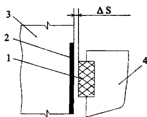
Рис. 28. Схема замера зазора в направляющих элементах линейно-подвижной опорной части:
