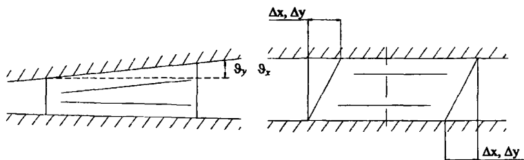
Рис. 24. Схемы обследования резиновых опорных частей
