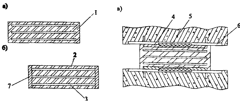
Рис. 8. Конструкции всесторонне-подвижных резиновых опорных частей:
