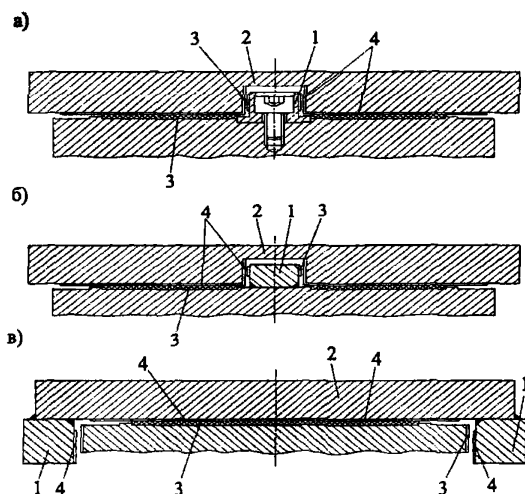
Рис. 6. Типовые примеры направляющих элементов:
