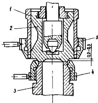
Рисунок Е.1 - Схема установки регулировочных втулок.
