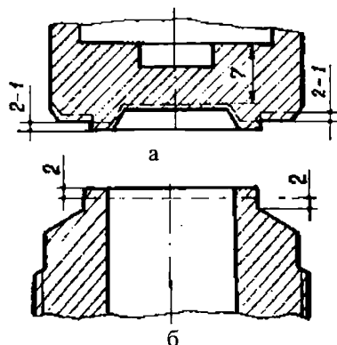
Рисунок Е.2 - Ремонтные размеры уплотнительных поверхностей: а – золотника; б – сопла
