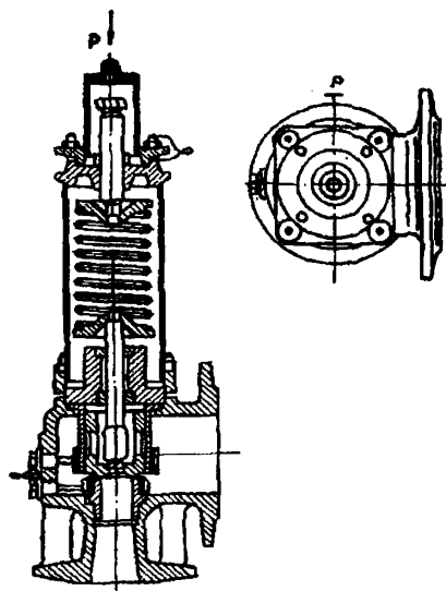
Рисунок И.6 - Клапан предохранительный пружинный типа СППК4 t до 600^{\circ}\text{C}
