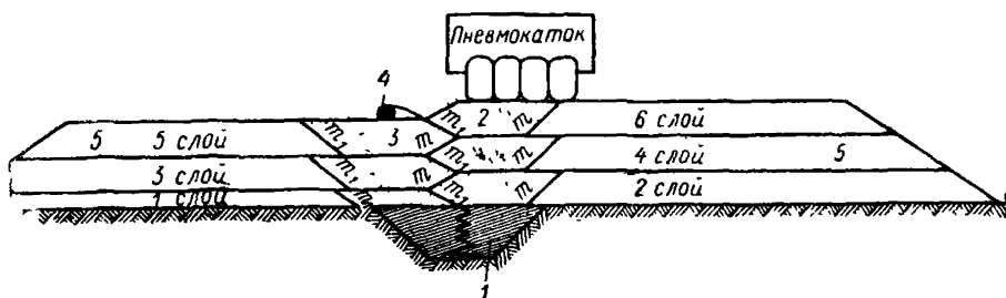
1-забивка зуба глиной, суглинком или бетоном, 2-подстилающий слой-песок, супесь, 3-защитный слой-супесь, песок, мелкая гравийка, 4-полиэтиленовая диафрагма-укладка рулонов при отсыпке шестого слоя, 5-тепло плотины из крупнообломочного материала, т-заложение, \frac{1}{2} соответствующее естественному откосу подстилающего слоя, \frac{1}{2} соответствующее естественному откосу защитного слоя.
