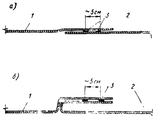
Рис. 7. Варианты соединений пленочных полотнищ
