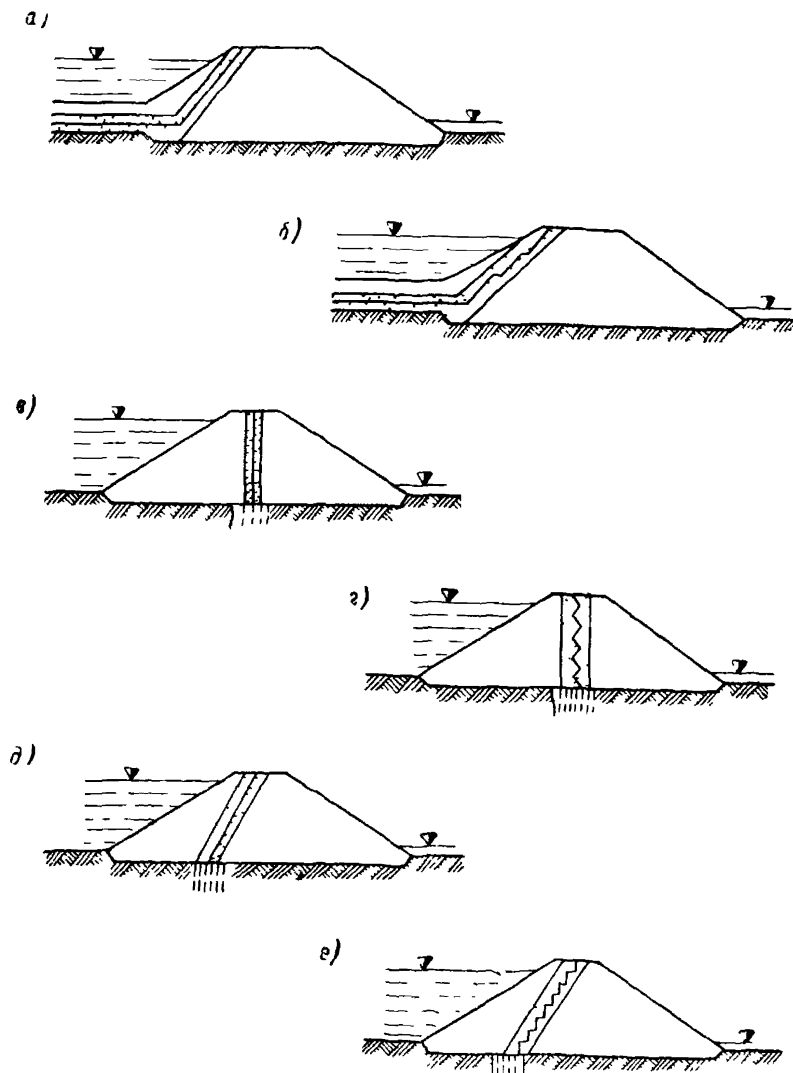
Рис. 1. Типы полиэтиленовых противофильтрационных устройств а—прямой экран и понур; б—ступенчатый экран и понур, в—прямая центральная диафрагма; г—ступенчатая центральная диафрагма, д—прямая наклонная диафрагма, е—ступенчатая наклонная диафрагма.
