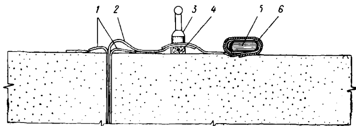
Рис. 10. Сварка рабочих полотнищ пленки на месте укладки 1—защитная пленка; 2—рабочая пленка; 3—импульсный полость; 4—подложка; 5—рулон; 6—защита рулона брезентом.
