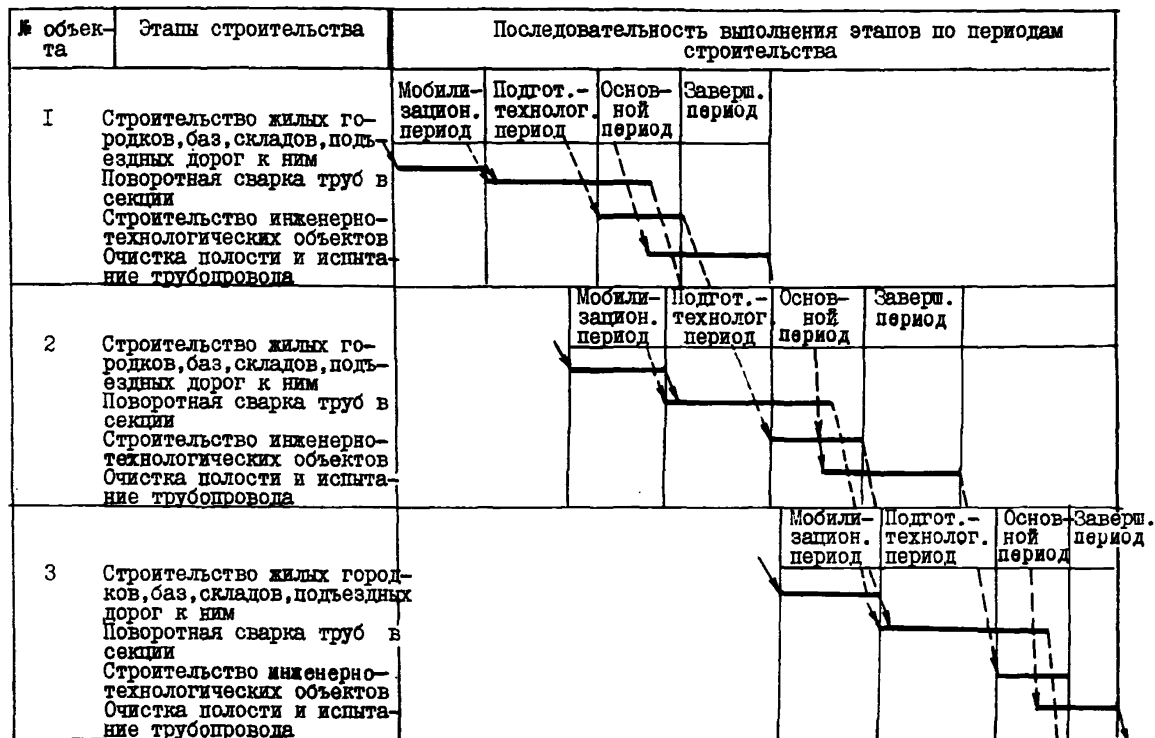
Рис.5. Схема поэтапной работы инженерно-технологического потока (ИТП) в составе межобъектного потока
