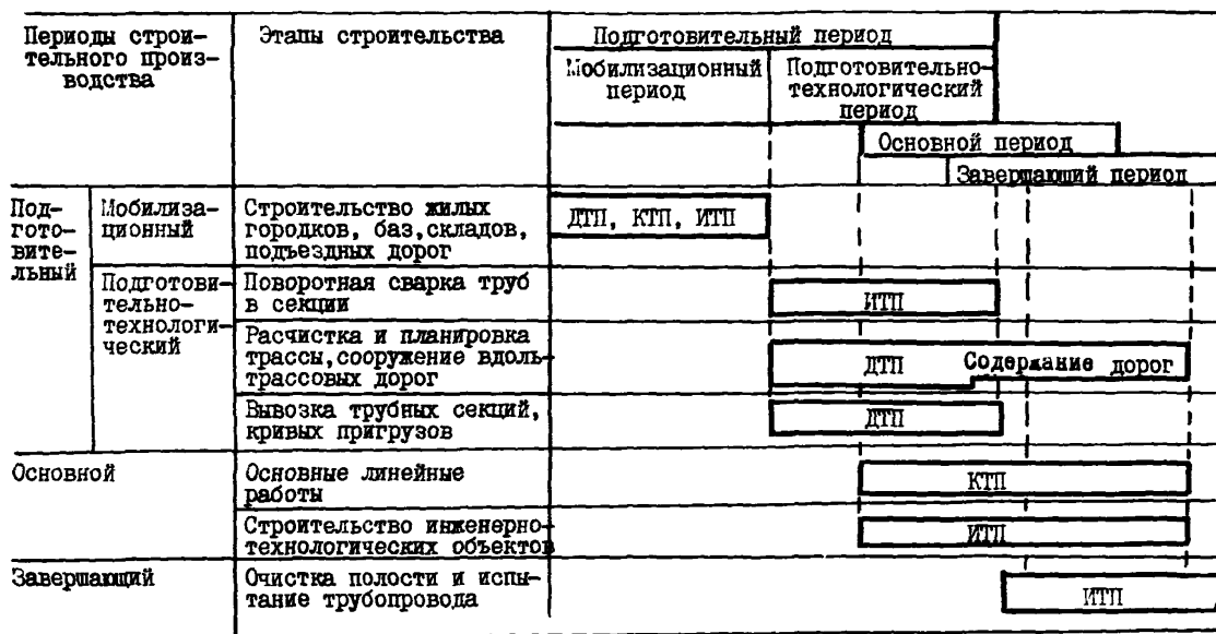
Рис. I. Схема распределения исполнителей и этапов трубопроводного строительства по периодам: Исполнители: ДТП – дорожно-транспортный поток; ИТП – инженерно-технологический поток; КТП – комплексный технологический поток
