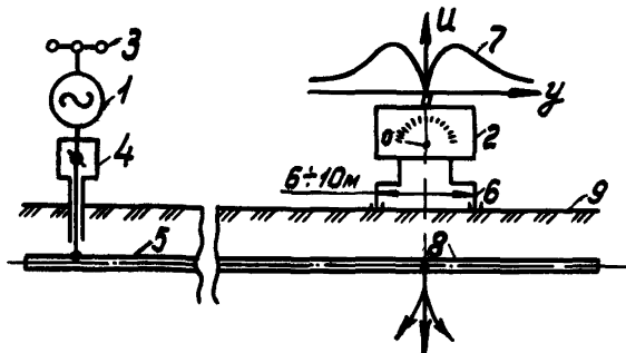
Рис. I. Схема поиска дефектов в изоляционном покрытии засыпанного одиночного трубопровода контактным продольным способом:
