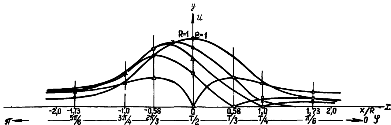
Рис.2. Изменение индуцированной в магнитной антенне электродвижущей силы в зависимости от горизонтального перемещения перпендикулярно трубе X и ориентации оси датчика \alpha относительно горизонтали.
