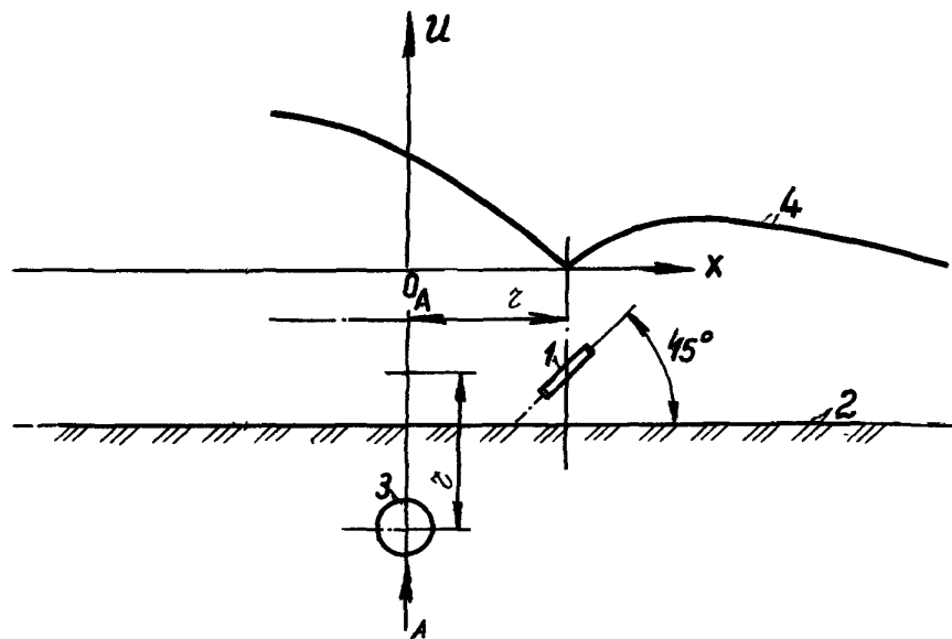
Рис.3. Определение глубины заложения трубопровода:
