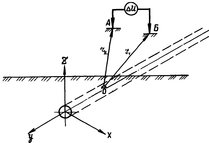
Рис.4. Схема определения дефекта в изоляционном покрытии:
