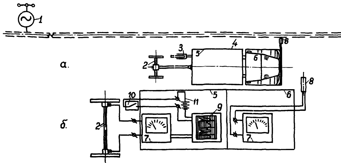
Рис.5. Схема механизированного поиска дефектов в изоляционном покрытии засыпанных трубопроводов:
