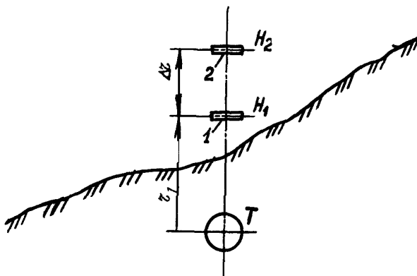
Рис.4. Определение глубины заложения трубопровода при наклонной поверхности земли:
