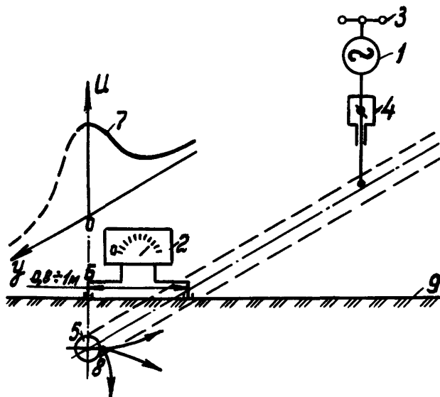
Рис.2. Схема поиска дефектов в изоляционном покрытии засыпанного трубопровода контактным поперечным способом (Обозначения даны на рис.1)
