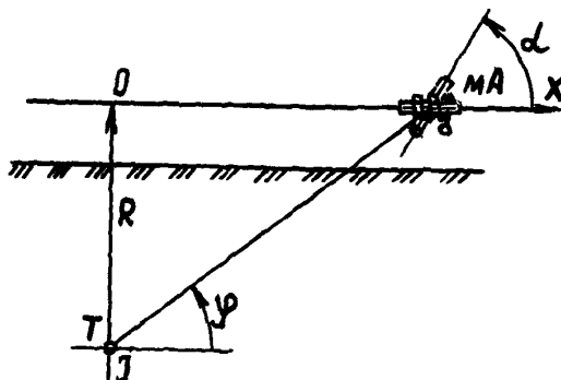
Рис. I. Взаимное расположение трубопровода Т с током I и магнитной антенны МА при определении трассы одиночного трубопровода:
