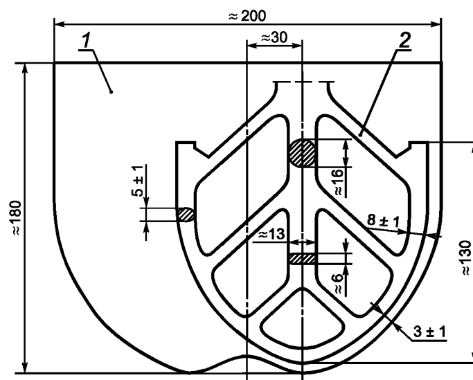
1 — чаша; 2 — лопасть
