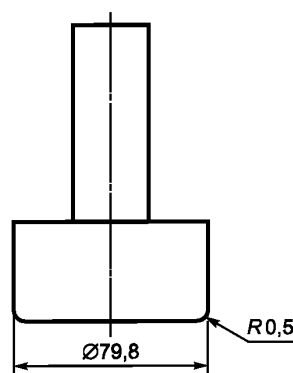
Рисунок 3 — Цилиндрический индентор
