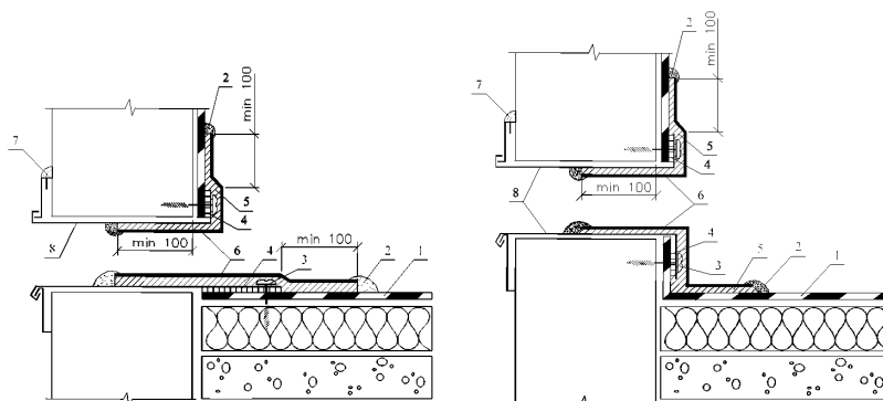
Рис Водотвод с кровли через parapet стену
