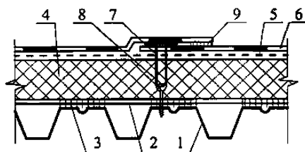
Рис Механическое крепление ПВХ мембраны ПЛАСТФОИЛ или
