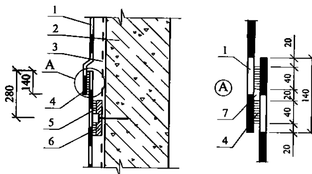
Рис Крепление полотенц ПВХ мембраны ПЛАСТФОИЛ или
