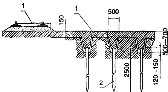
Рисунок 7 — Соединение заземлителей
