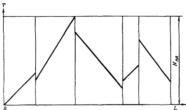
Рис.2. Топология директивного графика строительства трубопровода производственными комплексами при начале и окончании работ на отдельных участках в разное время
