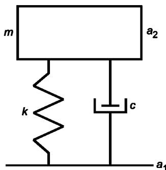
Рисунок А.1 — Система с одной степенью свободы
