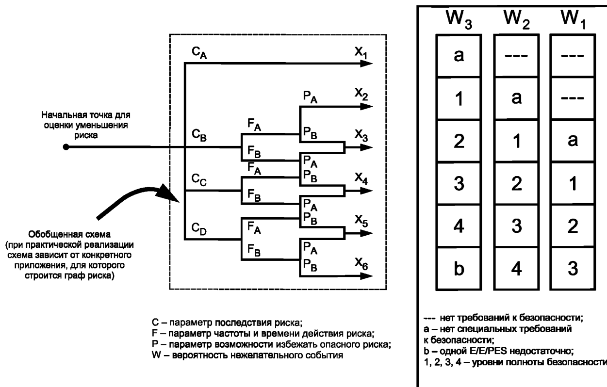
Рисунок D.1 — Граф риска: общая схема
