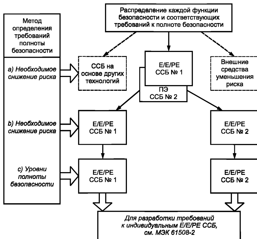
Рисунок А.3 — Распределение требований безопасности по Е/Е/РЕ системам, связанным с безопасностью, системам, связанным с безопасностью, основанным на других технологиях, и внешним средствам снижения риска
