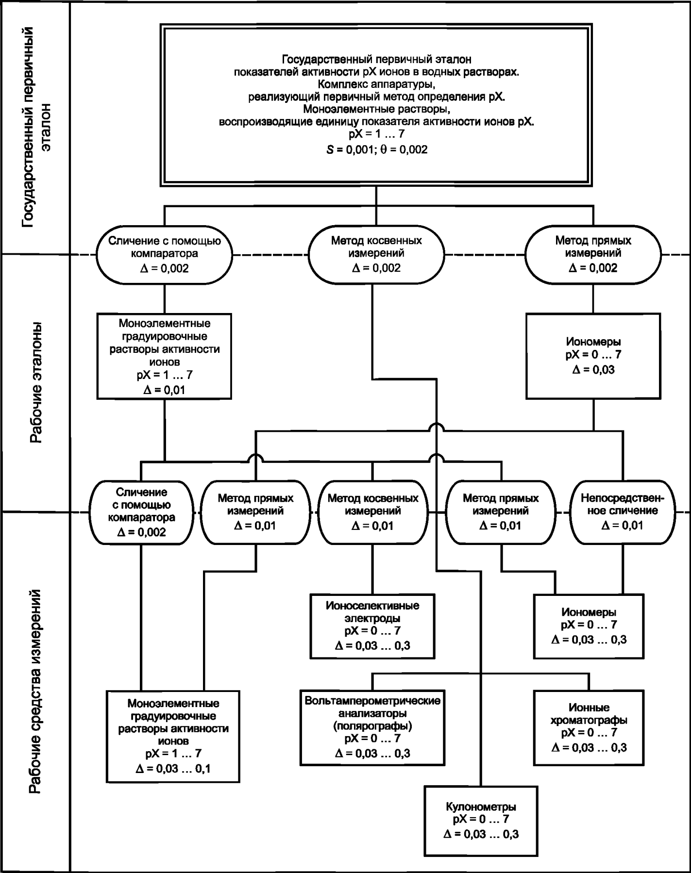
Государственная поверочная схема для средств измерений рХ
