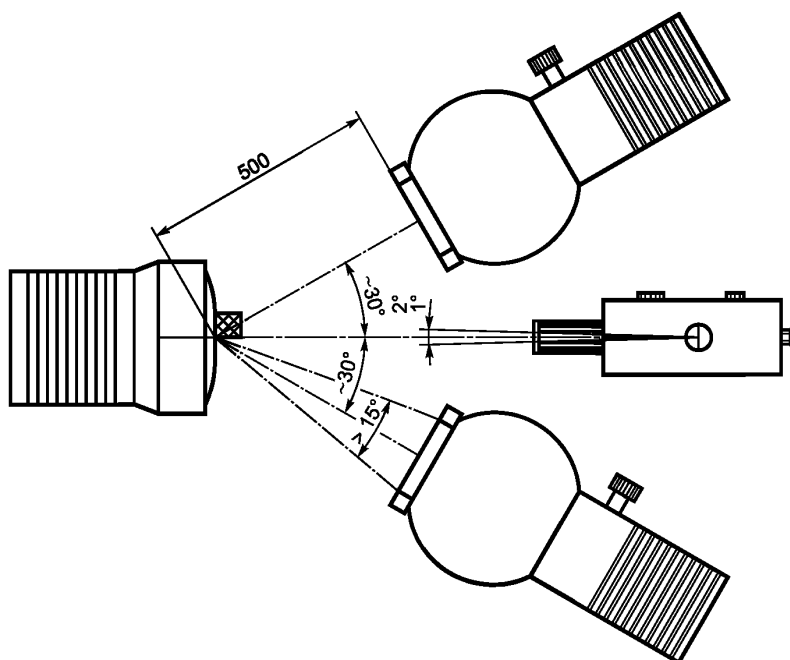
Рисунок 9 — Измерения диффузно отраженного излучения
