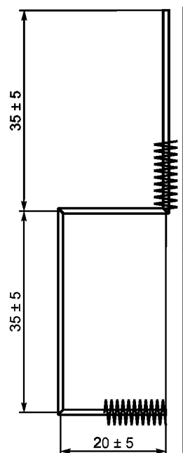
Рисунок 4 — Пример держателя для испытания на облуживание
