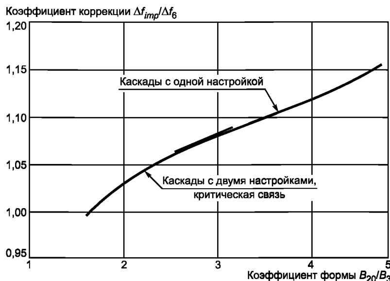
Рисунок Д.1 — Коэффициент коррекции для оценки отношения B_{imp}/B_6 для других типов настраиваемых схем
