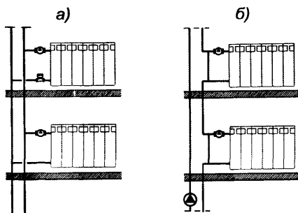
2.2. Схемы вертикальных систем отопления с радиаторами «FARAL Green HP» и «FARAL Green» а – двухтрубная, б – однотрубная
