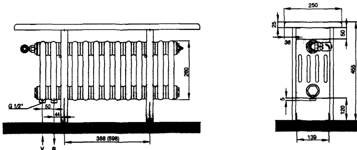
Рис. 1.7. Радиатор-скамейка «Zehnder Charleston Relax» модели CR 5026-13
