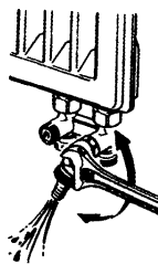
Рис. 5.5. Дренаж радиатора
