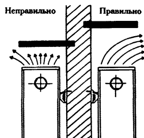
Рис. 5.4. Схемы установки радиатора под подоконником
