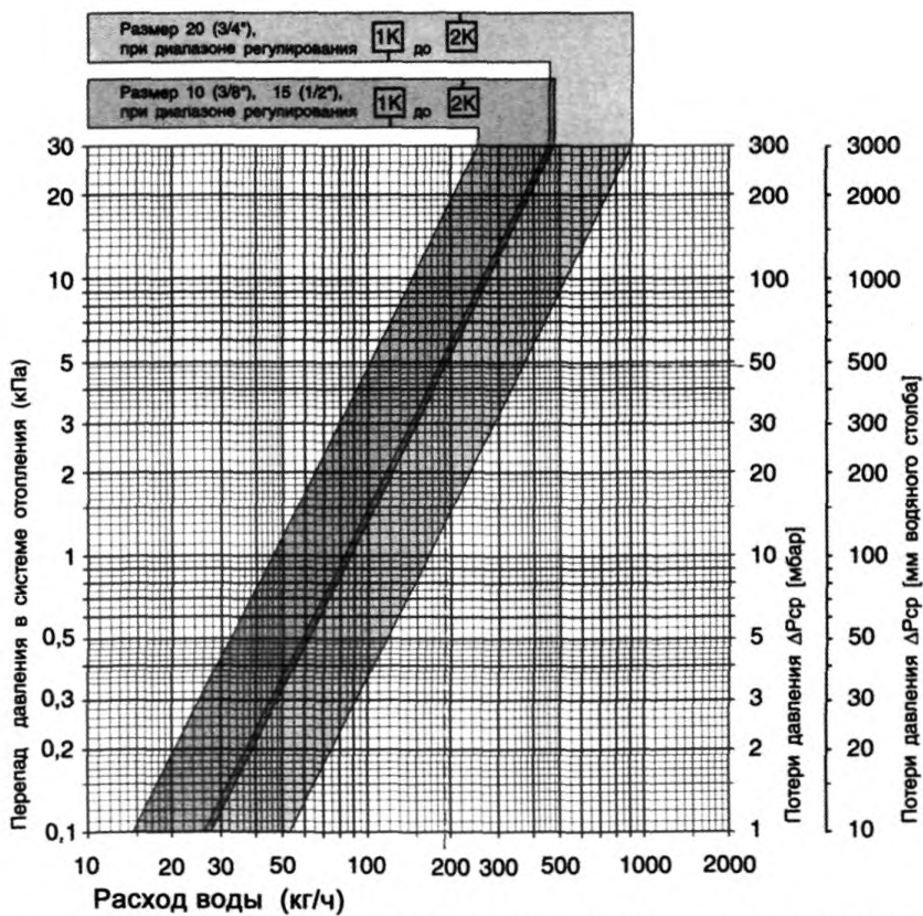
Рис. 2.4. Гидравлические характеристики термостатов «Super» фирмы «Heimeier»
