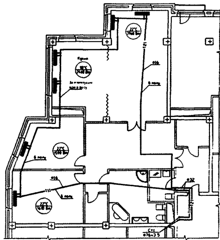
Рис. 1.7. Однотрубная поквартирная система отопления
