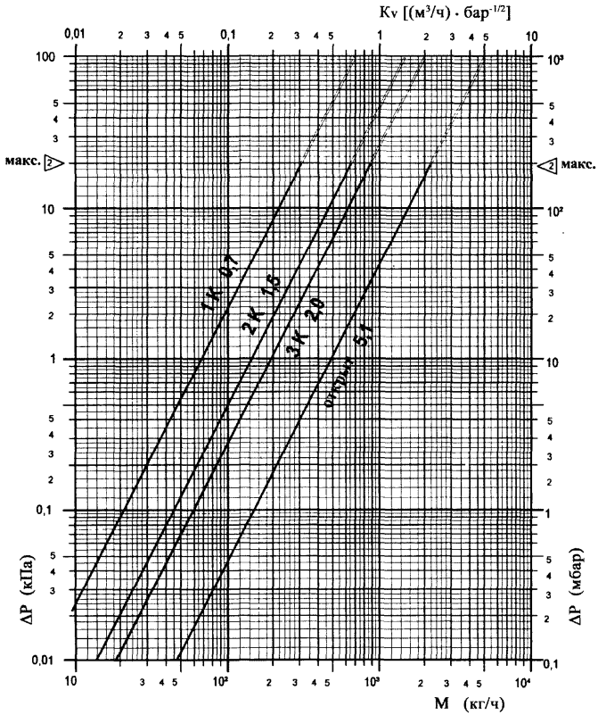
Рис. 3.2. Гидравлические характеристики термостатов «ГЕРЦ-TS-E» при различных режимах настройки
