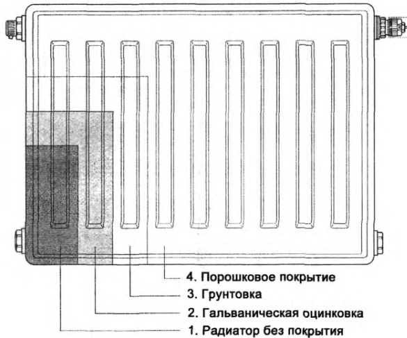
Рис. 1.3. Последовательность покрытия оцинкованных радиаторов «VONOVA»
