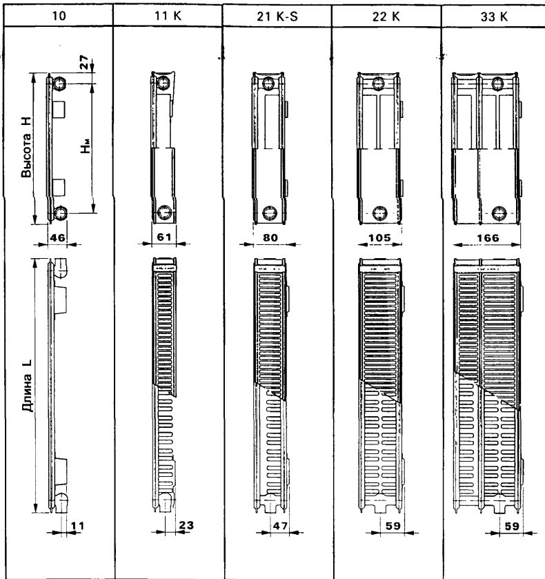
Рис. 1.2. Номенклатура радиаторов «VONOVA Компакт»
