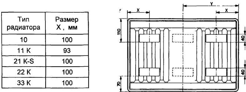
Рис. 6.1. Схема расположения скоб для крепления радиаторов всех типов на стене
