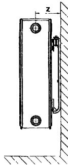
Рис. 6.1. Схема расположения скоб для крепления радиаторов всех типов на стене
