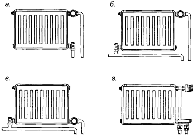
Ис. 2.2. Варианты присоединения радиаторов «VONOVA Kompakt» с термостатами фирмы «ГЕРЦ Арматурен» при напольной или плинтусной разводке теплопроводов
