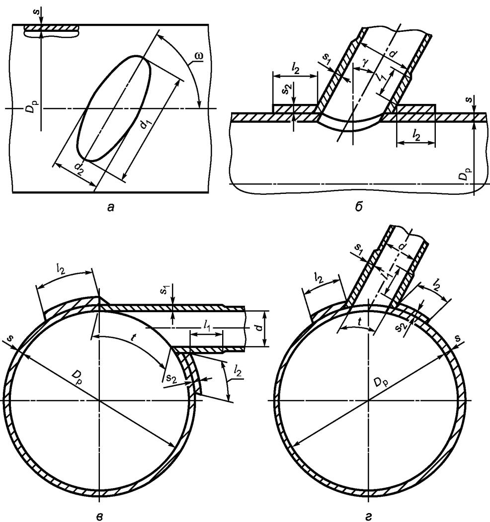
Рисунок А.11 — Наклонные штуцера на обечайке
