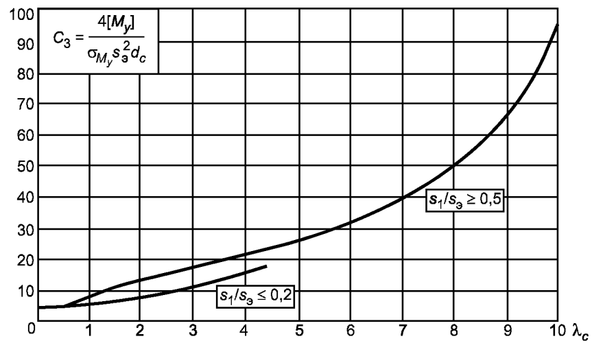
Рисунок А.18 — График для определения C_3
