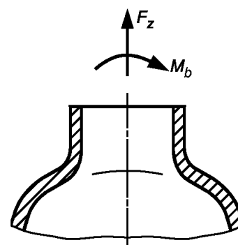
б — сферическое днище при внешних статических нагрузках на штуцер
