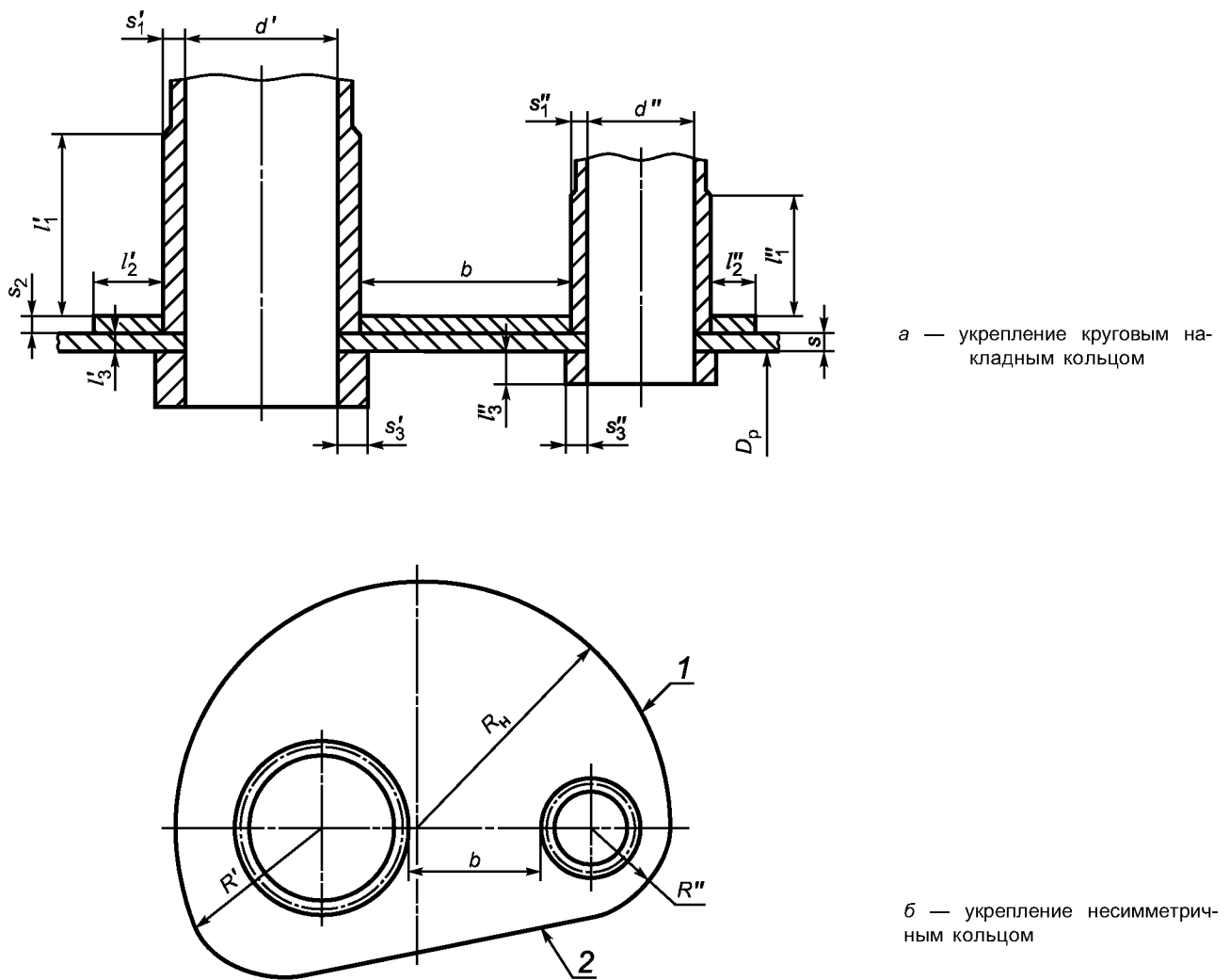
Рисунок А.8 — Совместное укрепление взаимовлияющих отверстий
