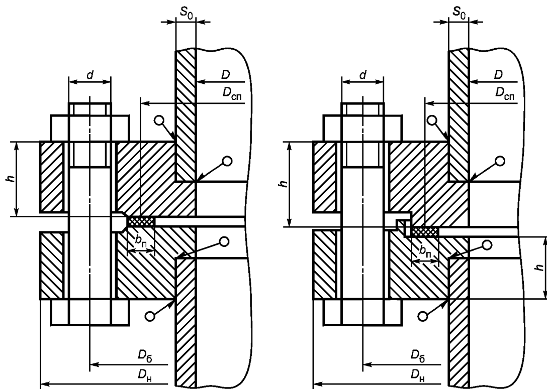
а — фланцевое соединение с гладкой уплотнительной поверхностью
