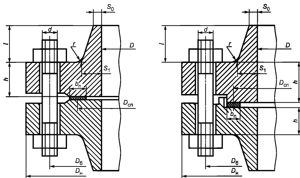
a — фланцевое соединение с гладкой уплотнительной поверхностью
