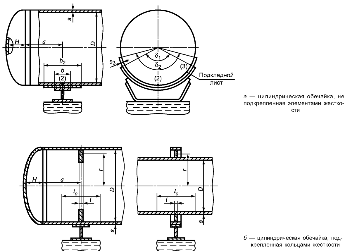
Рисунок 9 — Расчетная схема седловой опоры
