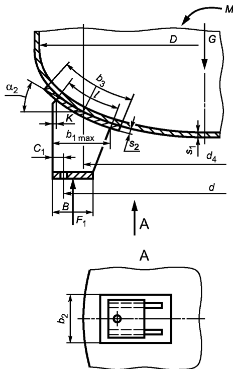
Рисунок 12 — Опорная стойка на эллиптическом днище
