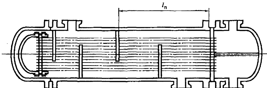
Рисунок 5 — Аппарат с плавающей головкой
