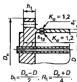
Рисунок 8 — решетка, приваренная встык к обечайке кожуха
