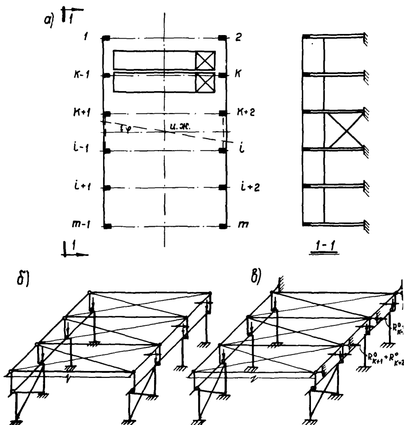
Рис.3.3. Расчетная схема каркаса при учете смещения от крановой нагрузки
