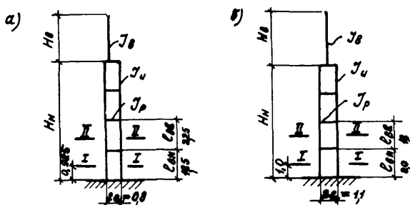
Рис.3.16. Схемы колонн а - крайнего ряда; б - среднего ряда
