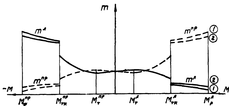
Рис. II. График зависимости момента в ветви m от момента в колонне M при наличии интервала значений M , в котором отсутствуют трещины в ветвях, т.е. при N \cdot e, > lq/kb
