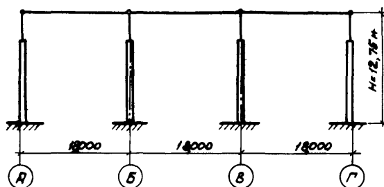
Рис.3.15. Расчетная схема рамы
