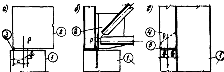
Рис.2.1. Схемы приложения вертикальных нагрузок P от стропильных конструкций и стен
