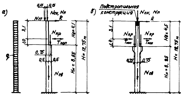
Рис.3.14. Схемы нагрузок на колонны а - крайнего ряда; б - среднего ряда
