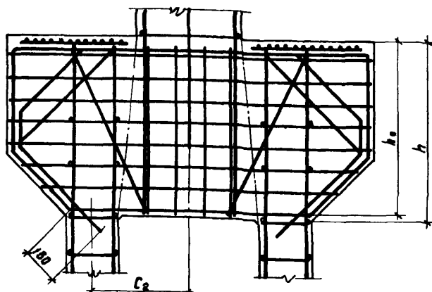
Рис. 4.16. Армирование верхней распорки крановой двух- ветвевой колонны среднего ряда
