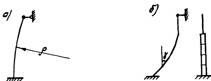
Рис.9. Схема изогнутой оси колонны а - при изгибе; б - при сдвиге
