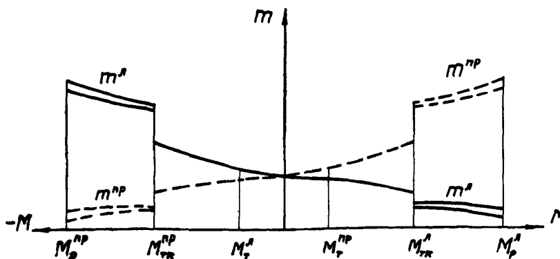
Рис. I2. График m-M при N \cdot e, \leq lq/kb
