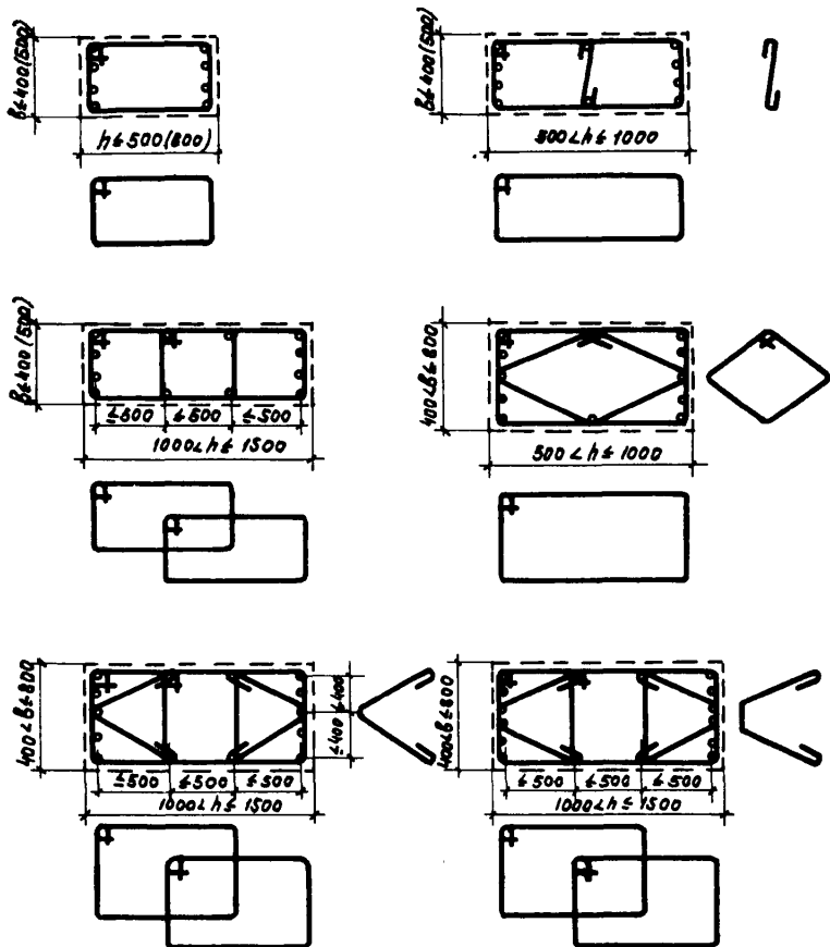
Рис. 4.6. Примеры конструкции вязанных каркасов колонн, вне- центрично сжатых в одной плоскости В скобках приведены размеры граней при толщине защитного слоя до продольной арматуры не менее 30 мм
