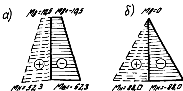
Рис.15. Эпюры моментов в колоннах при определении В экв.р.
