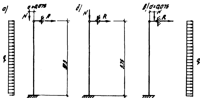
Рис.14. Схемы нагрузок на колонны а - по оси А; б - по осям Б, В, Г, Д, Е; в - по оси З
