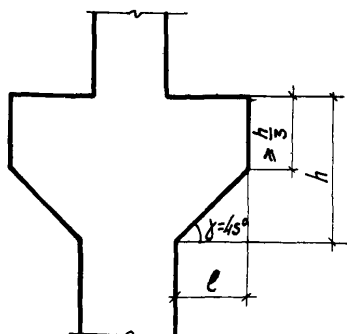
Рис. 4.10. Размеры подкрановой консоли h - не менее 200 мм и кратно 100 мм; l - не менее 200 мм, кратно 50 мм до 400 мм и далее кратно 100 мм
