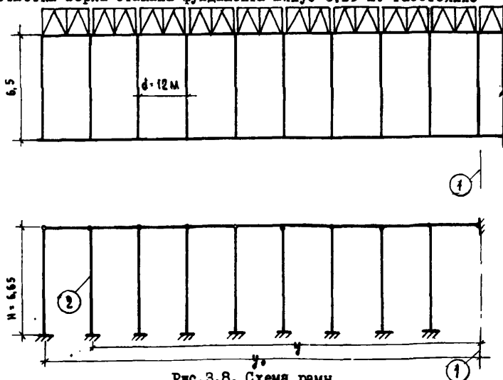
Рис.3.8. Схема рамы
