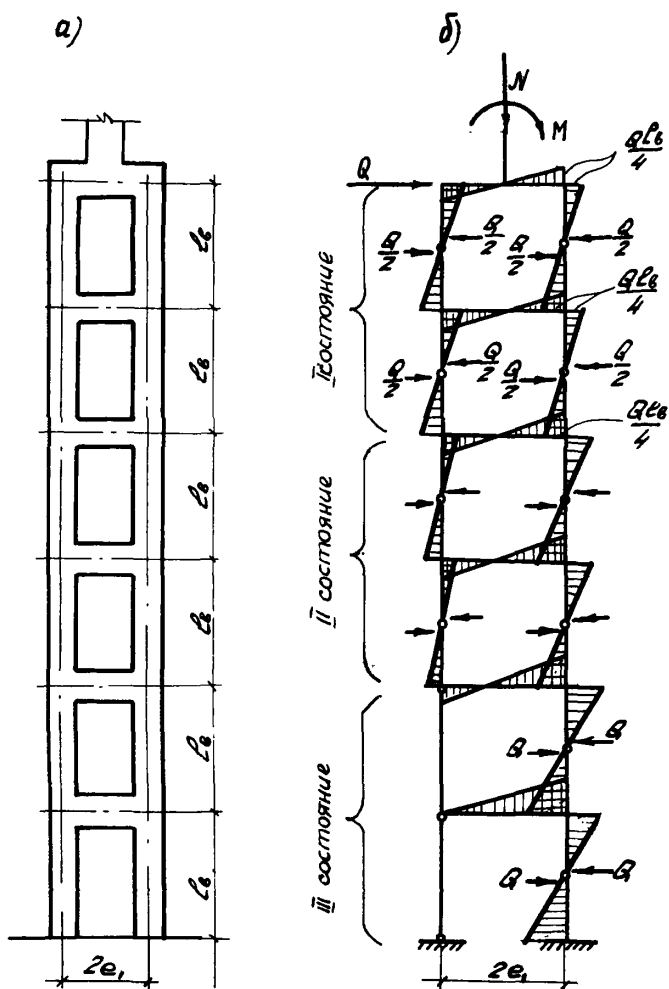
Рис.10. Схема двухветвевой колонны а - конструктивная; б - расчетная; I состояние - в ветвях отсутствуют трещины; II состояние - в левой ветви есть трещины, обе ветви сжаты; III - состояние - левая ветвь растянута
