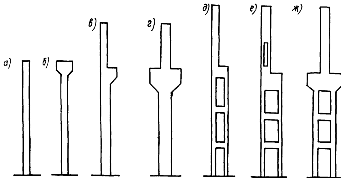
Рис. I, 5. Типы колонн
