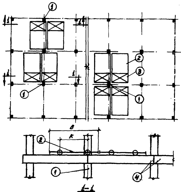
Рис.2.2. Схемы неблагоприятного расположения мостовых кранов
