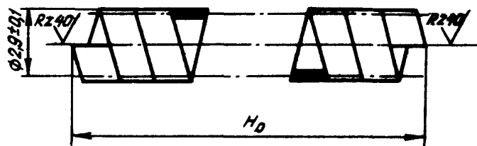
Развертка М5:1
