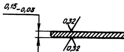
Сечение витка М20:1
