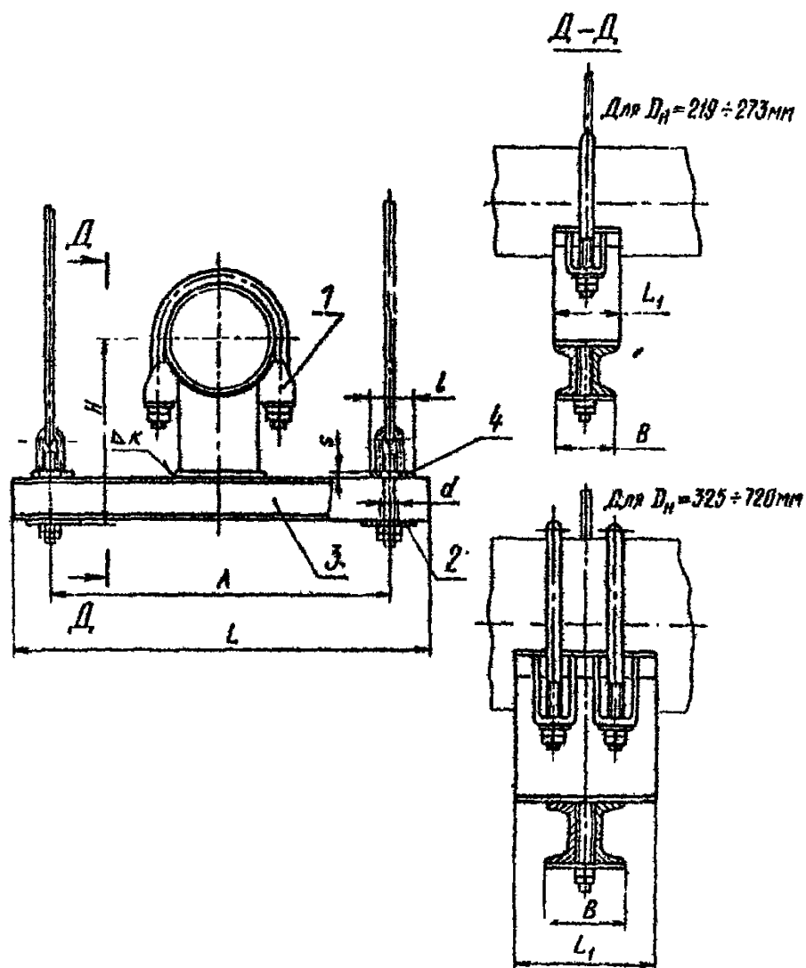
1 — опора; 2 — плита опорная; 3 — балка опорная; 4 — планка
